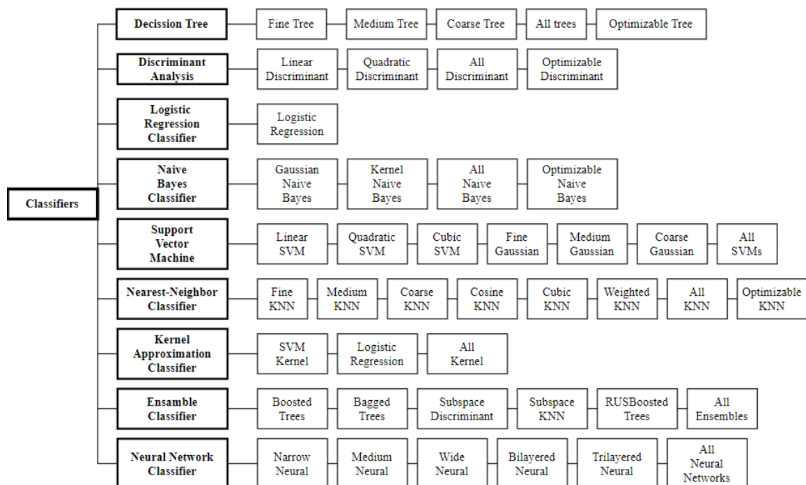
Obrázek 5.1: Klasifikátory, které byly testovány, upraveno z [59]
