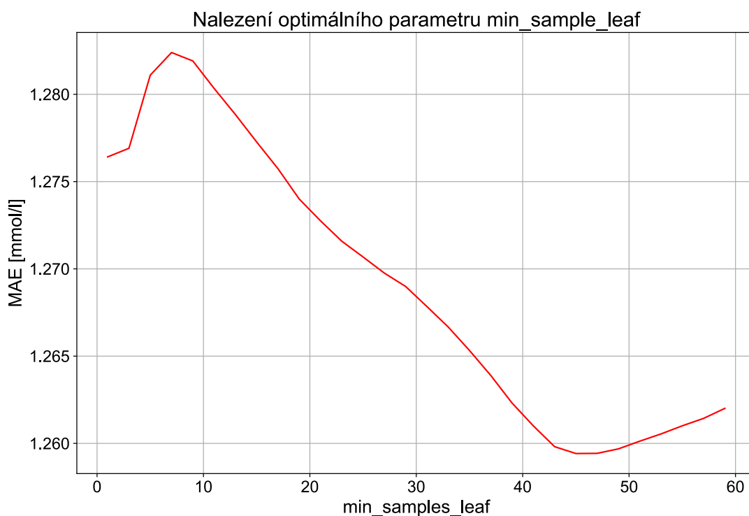
Obrázek 9.11: Nalezení optimálního počtu parametru min samples leaf pro regresi (23 příznaků)
