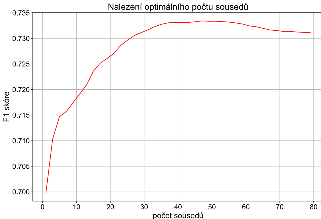
Obrázek 9.1: Optimální počet sousedů (10 příznaků)
