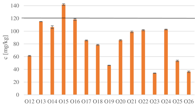
Obrázek 13: Koncentrace zinku ve vzorcích z Ostravy
