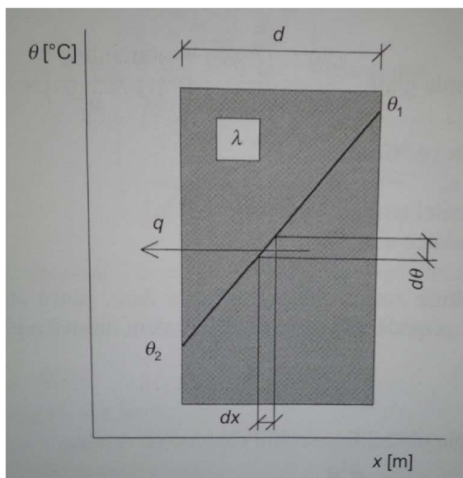
Obr. 3.1 Sdílení tepla vedením. [3]
