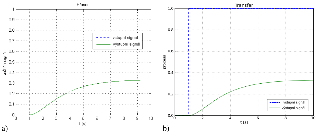
Obr. 5 – Průběh jednotkového skoku přes řízený systém. a) V Simulinku. b) V tomto programu.
