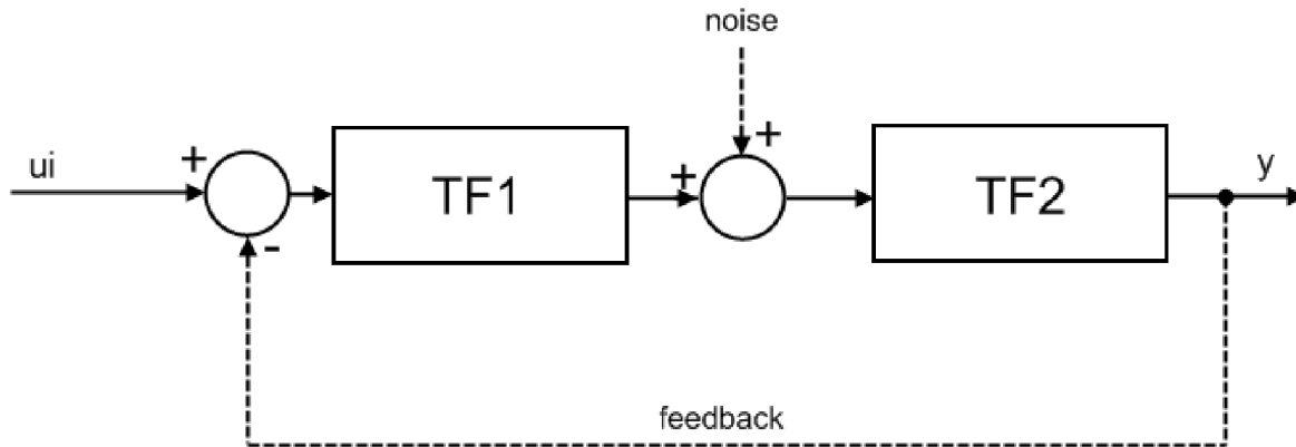
Obr. 3 – Znáznornění funkce transfer
