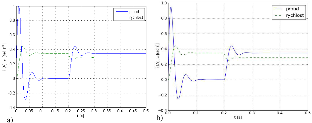
Obr. 13 – Rozběh stejnosměrného motoru. a) V Simulinku. b) V tomto programu.
