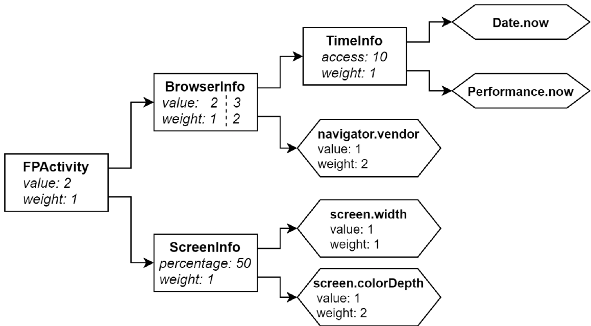
Obr. 4.1: Príklad heuristik, ktoré je možné definovať konfiguračnými súborami modulu Fingerprinting Detection. Obdĺžniky predstavujú príklady skupín zo súborov groups-lvl_X.json . Šesťuholníky predstavujú príklady obalovaných prostriedkov zo súborov wrappers-lvl_X.json .
