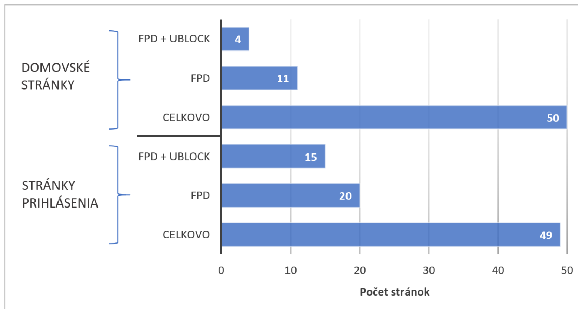
Obr. 5.11: Porovnanie počtu detekcií pri samostatnom použití rozšírenia JavaScript Restrictor s modulom Fingerprinting Detection (FPD) a kombinácií tohto rozšírenia s nástrojom uBlock Origin . Testovanie bolo vykonávané na domovských stránkach a aj na stránkach prihlasovania. Celkový počet stránok prihlasovania je nižší, pretože nie všetky stránky umožňujú prihlásenie užívateľa.
