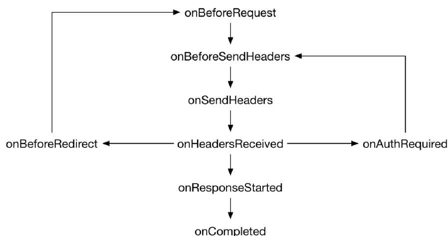
Obr. 3.4: Udalosti reprezentujúce jednotlivé fázy spracovania HTTP požiadavky. Prevzaté z [28].
