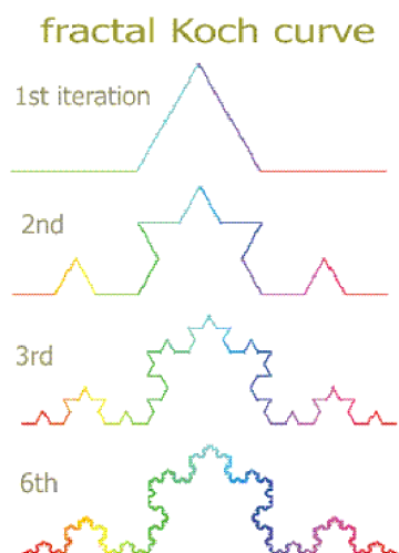
Obrázok 1: Kochova krivka
