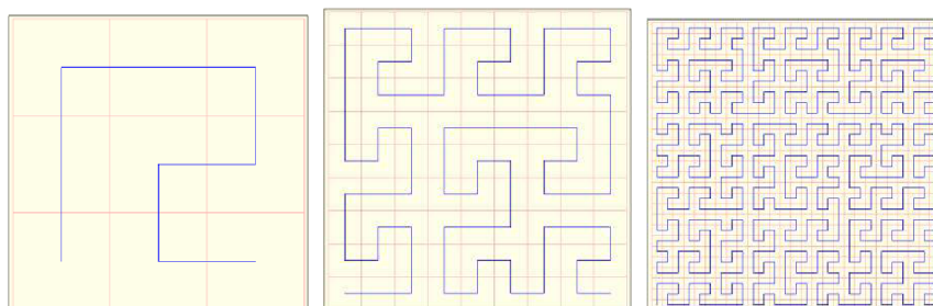
Obrázok 8: Wunderlichova krivka 3
