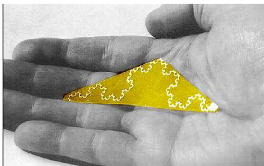
Obrázok 20.: Fraktálna anténa
