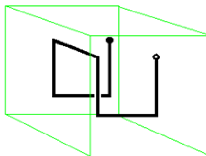
Obrázok 14.b: Základná Hilbertova 3D krivka pri pohľade spredu.
