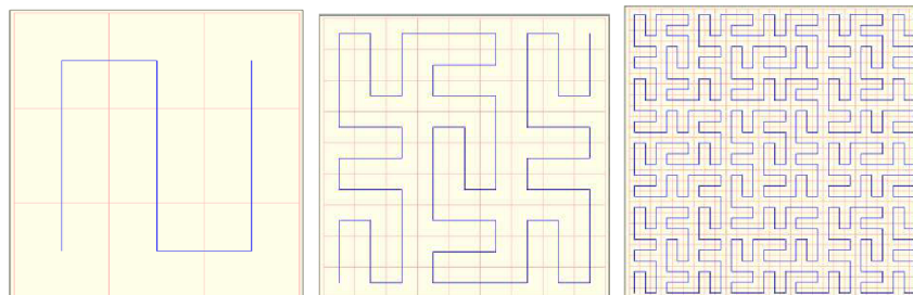
Obrázok 7: Wunderlichova krivka 2
