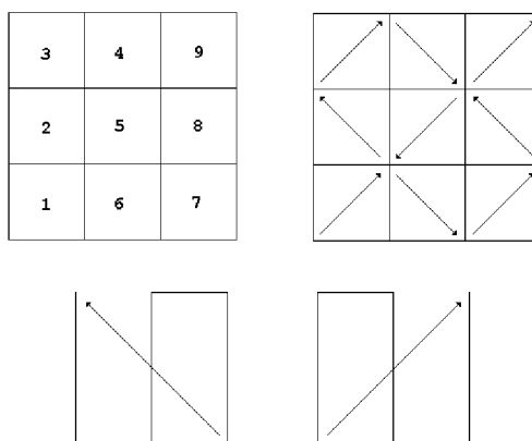
Obrázok 4: Tvorba Peanovej krivky
