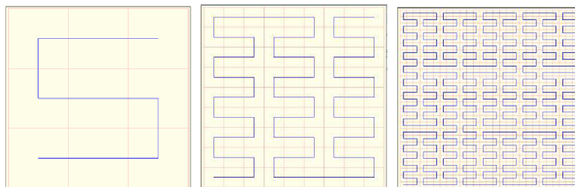
Obrázok 6: Wunderlichova krivka 1
