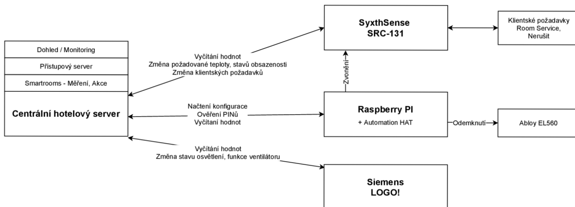
Obr. 7.3: Schéma komunikace jednotek v pokoji s jednotkou SyxthSense SRC-131
