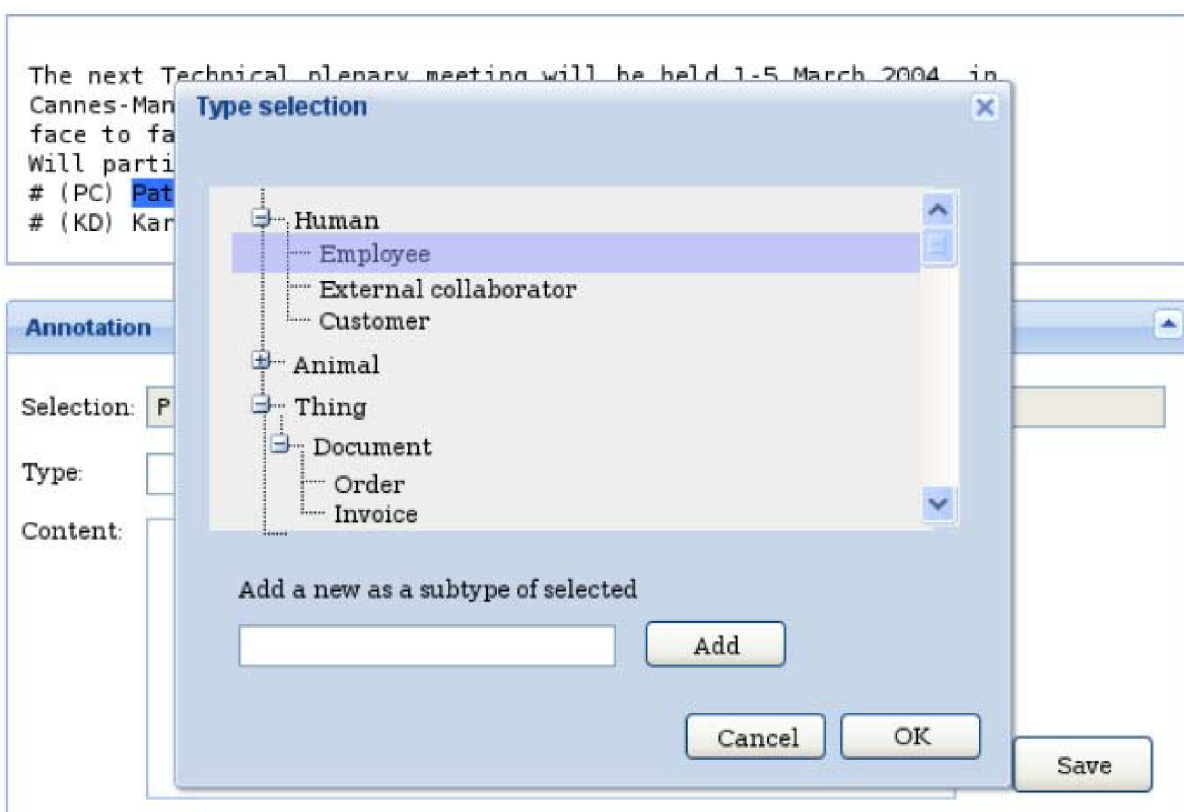
Obrázok 13: Výber typu zo stromu typov [47].
