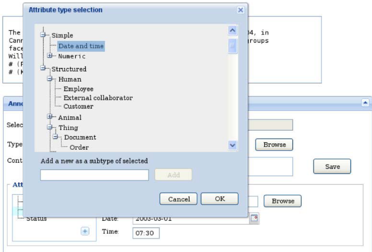
Obrázok 14: Výber typu atribútu zo stromu typov [47].
