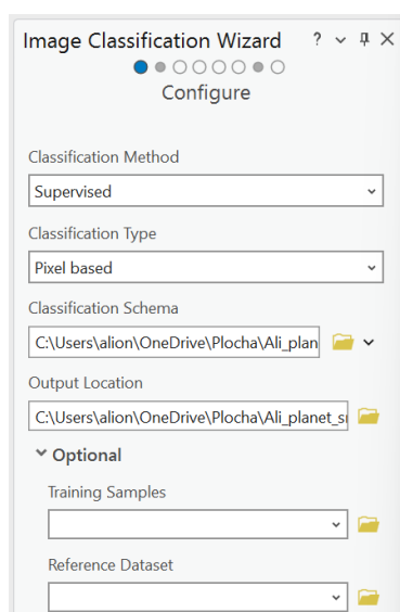
Obrázek 15: Použité nastavení nástroje Classification Wizard – Configure
