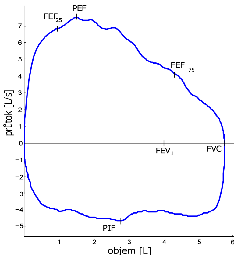
Obrázek 2: Křivka průtok-objem.
