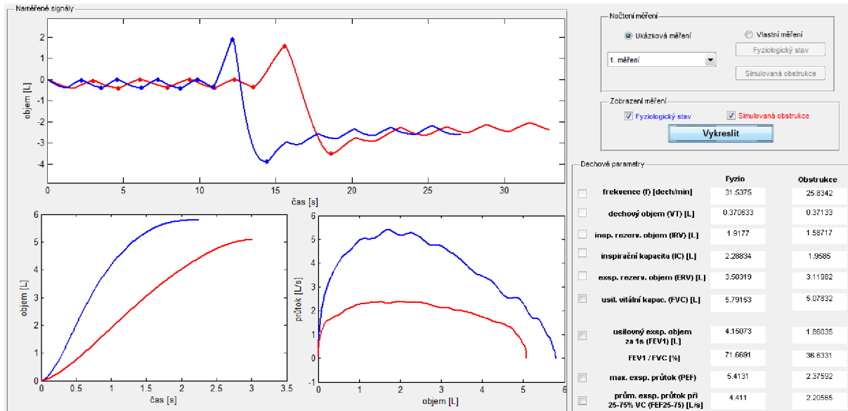
Obrázek 10: Programové okno.
