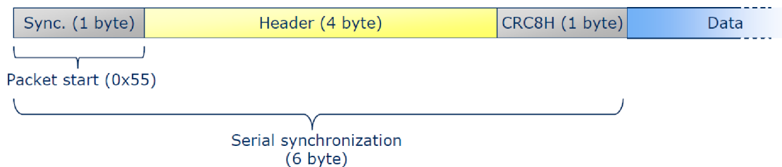
Obr. 20: Ukázka synchronizační části paketu [25]
