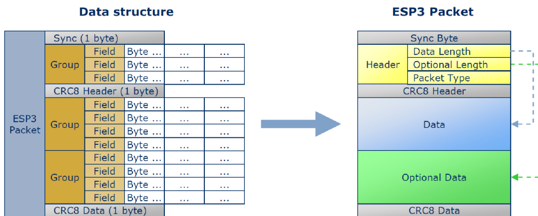
Obr. 17: Struktura paketu [25]
