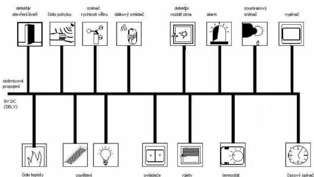
Obr. 3: Princip propojení zařízení u sběrníkového systému elektroinstalace [3]
