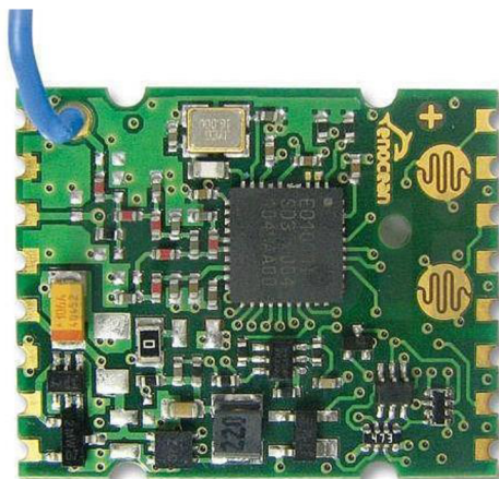
Obr. 10: Bezdrátový modul EnOcean PTM 332 [18]
