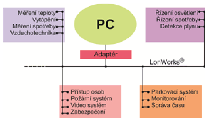
Obr. 7: Příklad systému LonWorks [12]
