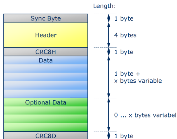
Obr. 18: Znáornění délky paketu [25]
