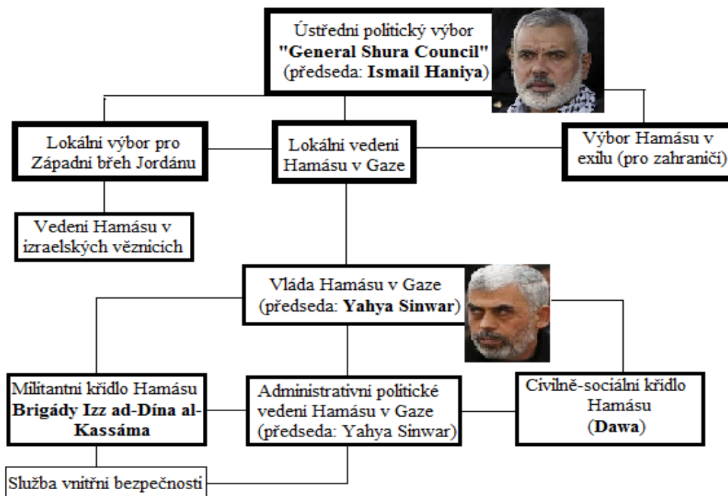
Obrázek 3: Struktura Hamásu
