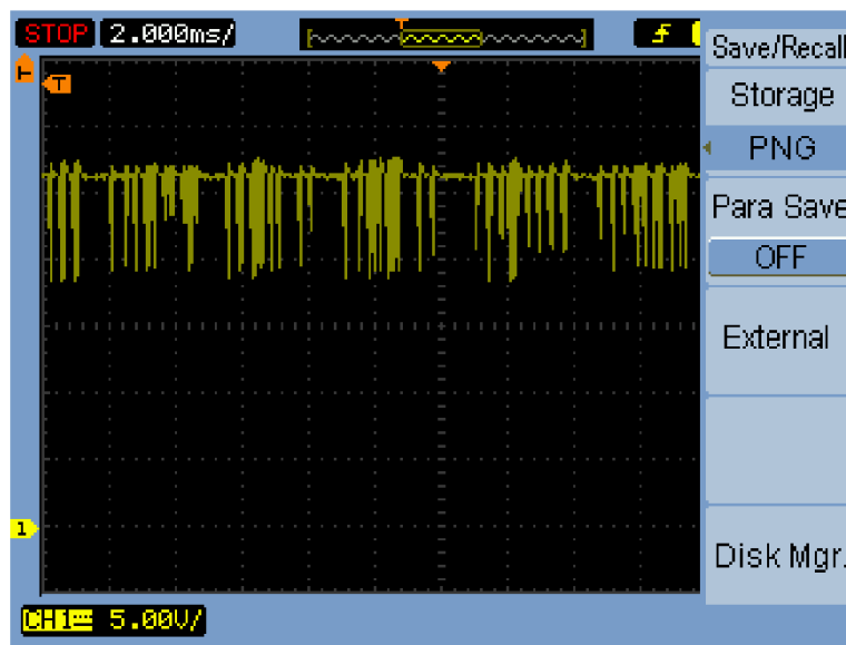
Obr. 4-5 Přenos dat na sběrnici CIB
