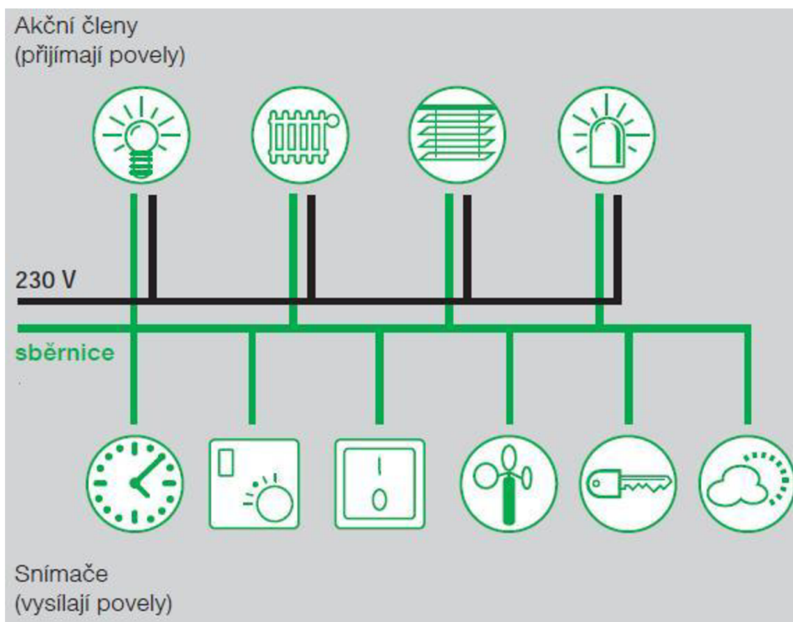
Obr. 1-2 Moderní sběrnicevých elektroinstalací[2]
