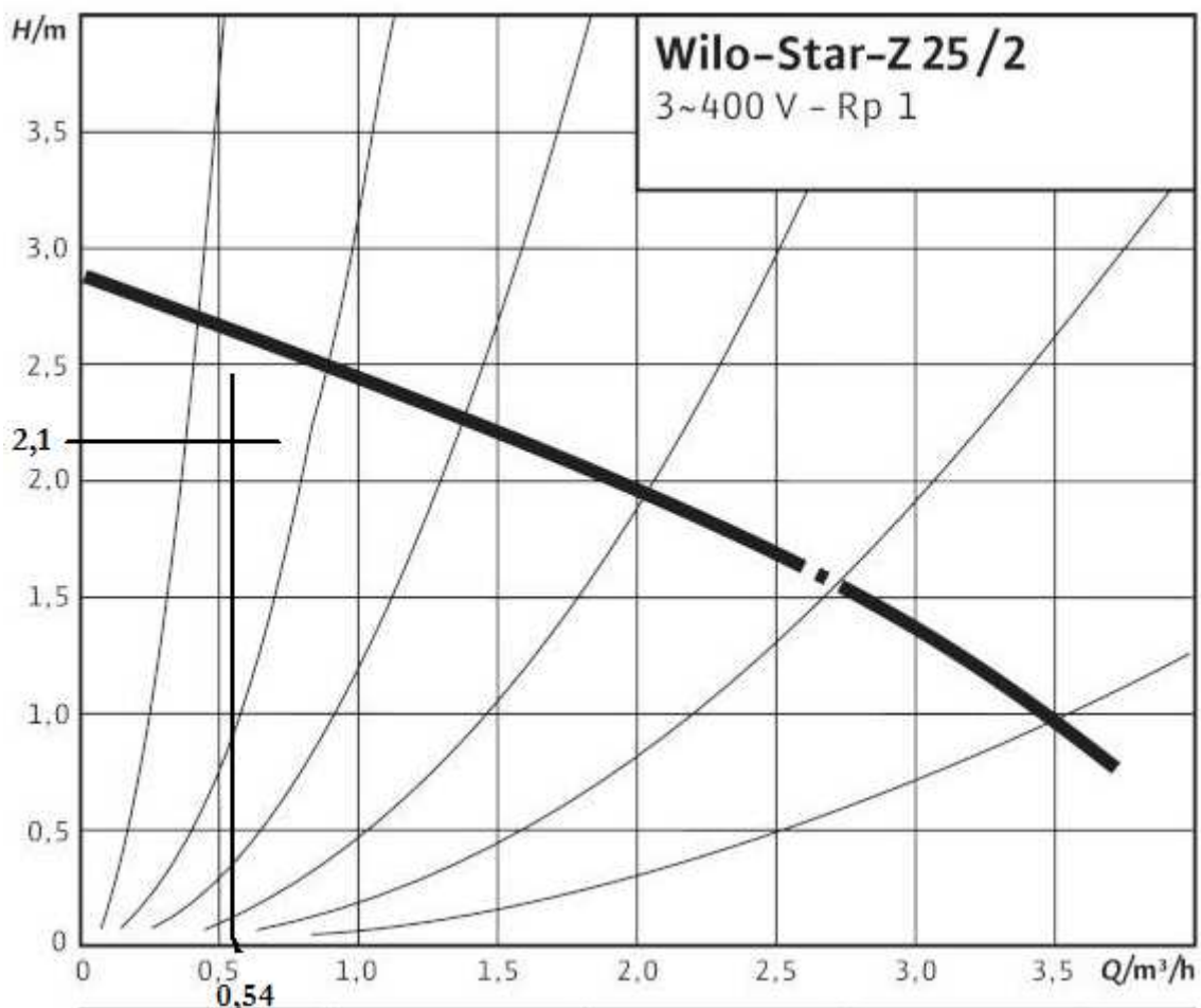
Obr. 30: Charakteristika čerpadla [11]
