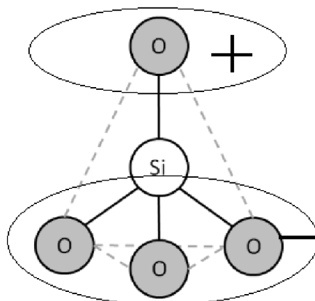
Obr. 8: Znáornění vzniku částečných nábojů v důsledku působení mechanické deformace. Převzato a částečně upraveno. [27]
