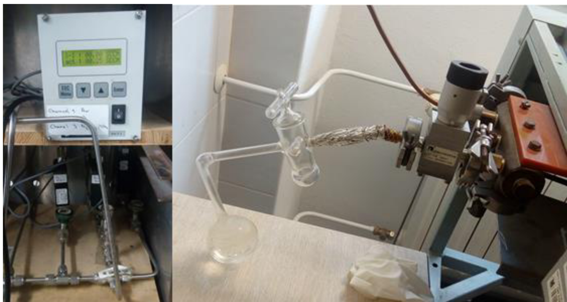
Obr. 13: Na levém obrázku je řídicí jednotka průtokoměrů a na pravém obrázku je způsob dávkování monomeru CPA bez izolace baňky s vodní lázní.
