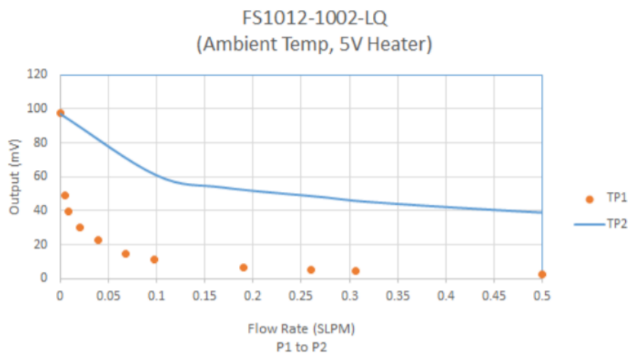
Obr. 3-6 Závislost napětí na průtoku deklarovanou výrobcem u senzoru FS1012-1002-LQ [5]
