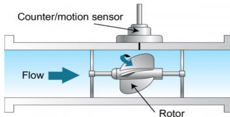
Obr. 1-4 Turbínový rychlostní průtokoměr. Průtok (flow) je hnán přes rotující část (rotor), kterou snímá otáčkoměr (counter sensor) nebo pohybový senzor (motion sensor). [19]
