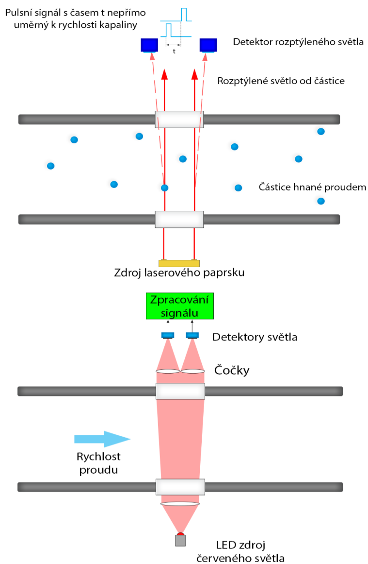
Obr. 1-7 Nahoře optické senzory na principu L2F a dole princip scintilace.
