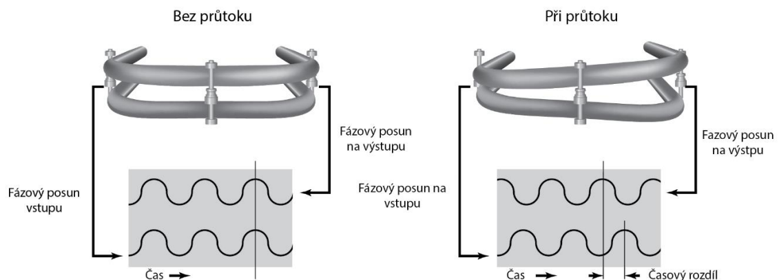
Obr. 1-7 Znárodnění Coriolisova principu. V První části bez průtoku je fáze stejná v druhé části je již průtok přítomen a fáze se posunuje. [20]
