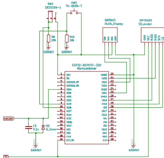
Obr. 3-11 Zapojení periferií do ESP32 DevKit 32D
