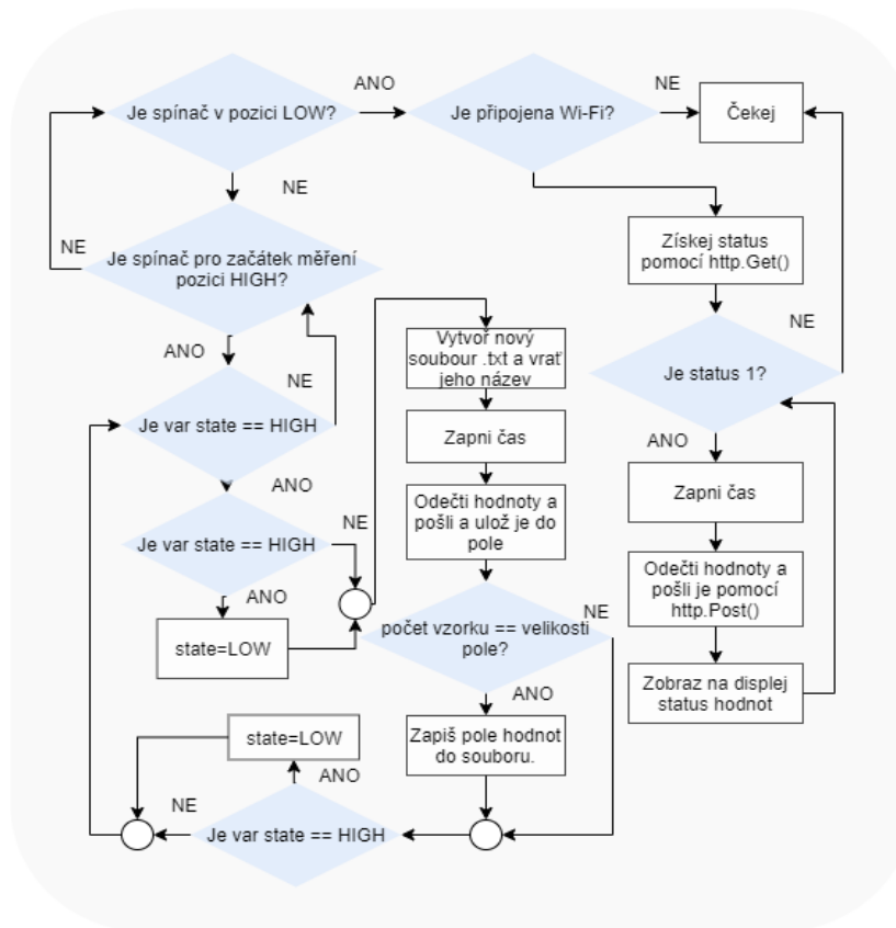
Obr. 4-5 Diagram s algoritmizací funkce loop()
