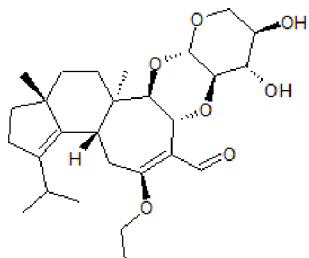
Erinacin D
