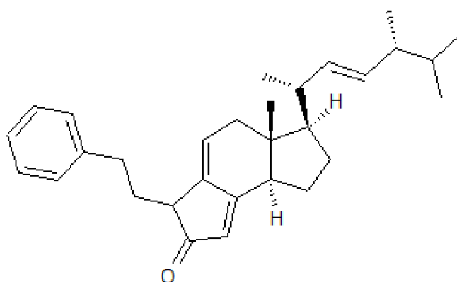
Hericin
