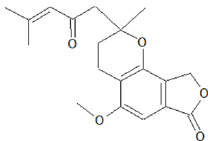
Hericenon I
