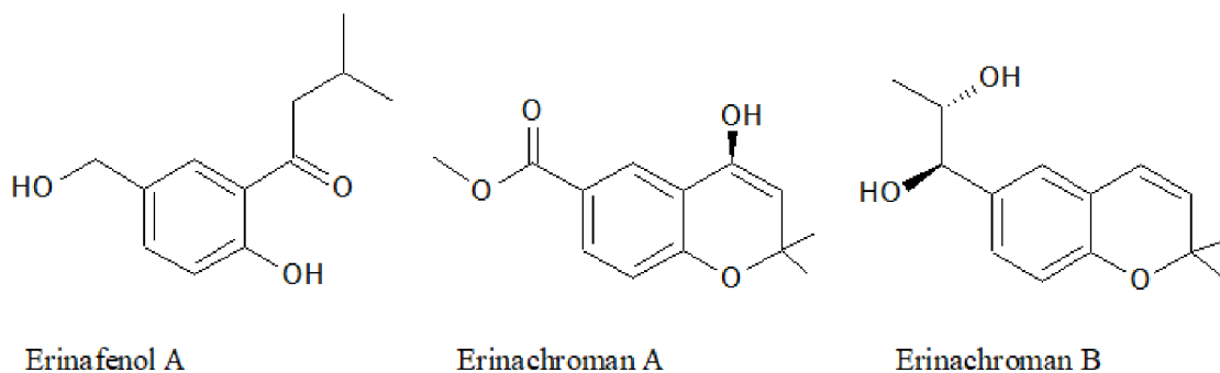
Obrázek 12: Chemická struktura erinafenolu A a erinachromanů A-B
