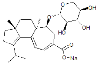
Erinacin H
