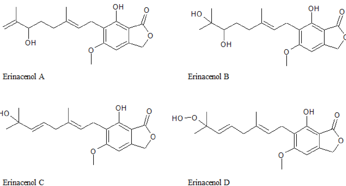
Obrázek 20: Chemická struktura erinacenolu A-D
