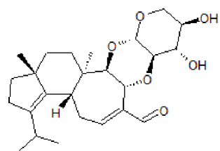
Erinacin B
