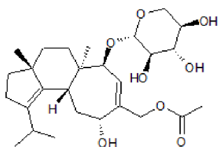
Erinacin K
