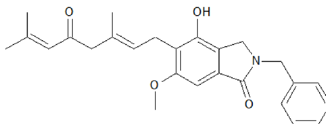
Hericenon B
