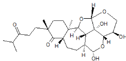
Erinacin J
