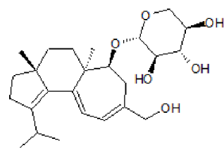
Erinacin C
