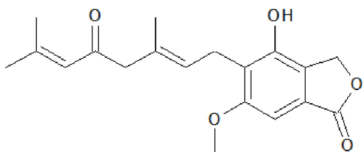
Hericenon A
