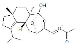
Erinacin G
