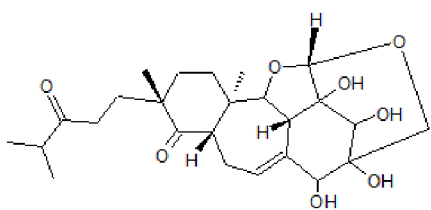
Erinacin G
