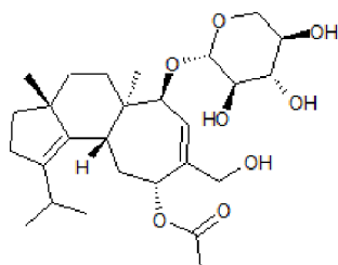
Erinacin Q
