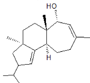
Erinakol
