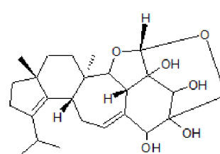
Erinacin F
