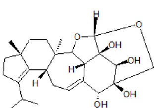
Erinacin E
