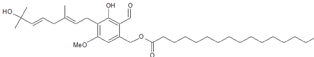
Erinacen D
