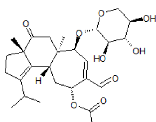
Erinacin R
