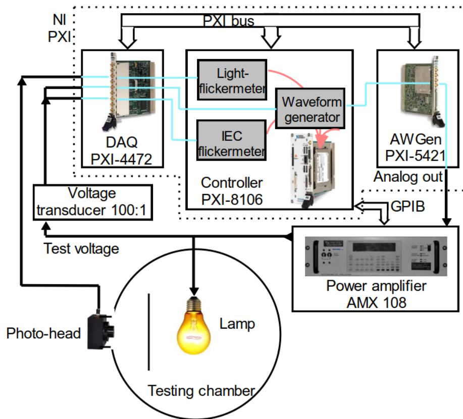
Obr. 4-3 Blokové schéma testovacieho pracovišťa [4]
