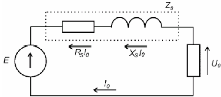
Obr. 3-2 Jednofázový náhradní obvod napájecí sítě [3]
