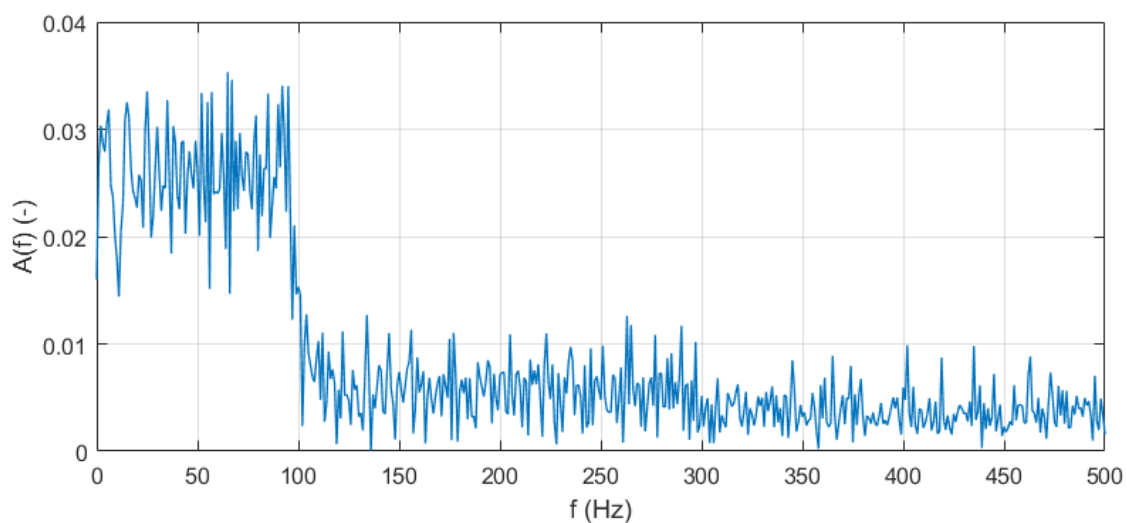
Obr. 6-24 Frekvenční amplitudové spektrum výsledného signálu
