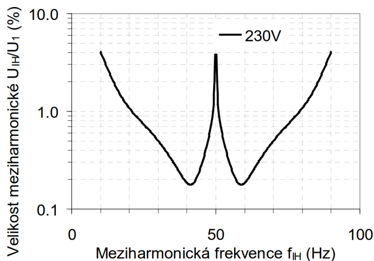
Obr. 2-3 Kompatibilní úroveň pro meziharmonická napětí související s blikáním referenční 60 W žárovky jako funkce meziharmonické frekvence do 100 Hz [2]
