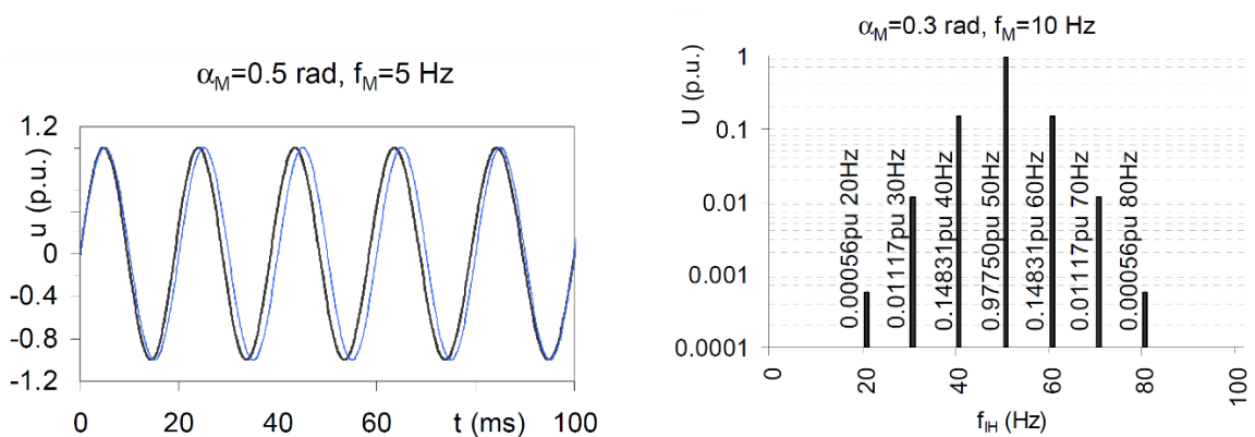
Obr. 3-8 Fázová modulace (PM) – sinusový modulační signál [1]
