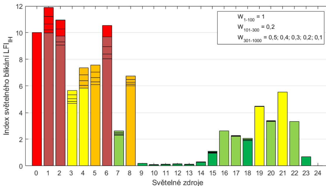
Obr. 6-7 Graf indexů LFI_{IH} pro různé hodnoty W_{301-1000}
