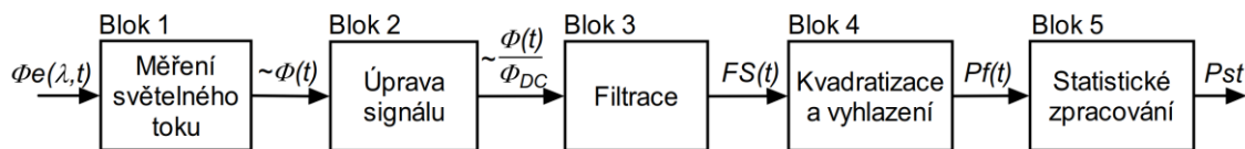
Obr. 4-2 Blokové schéma objektivního flickrmetru [2]
