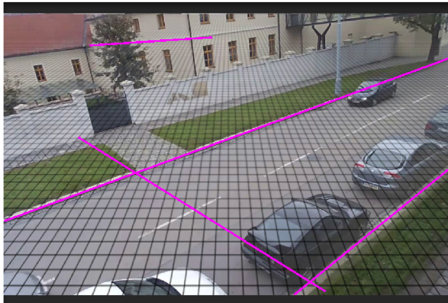
Obrázek 4.7: Poloaautomatická kalibrace. Viditelné jsou dvě sady přímek, které na sebe jsou ve skutečném světě kolmé. Dvě přímky podél silnice jedna osa (nejčastěji Z), zbývající dvě jsou kolmé na ty první. Všimněte si rozmístění přímek, zvláště druhého páru – čím větší je na obrazovce úhel mezi rovnoběžnými přímkami, tím je výsledek přesnější
