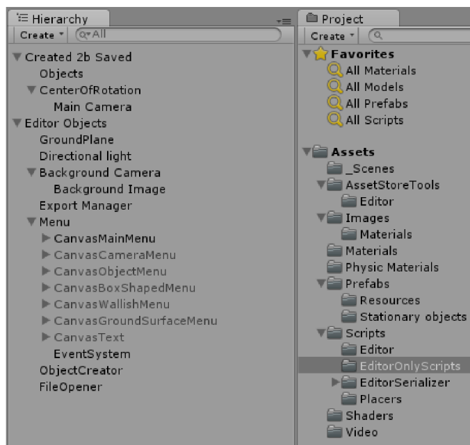
Obrázek 4.1: Struktura projektu v Unity Editoru. Hierarchie GameObjectů nalevo, hierarchie assets napravo. Zašedlé objekty jsou neaktivní.
