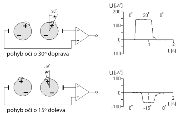
Obr. 3.1: Princip EOG [14]
