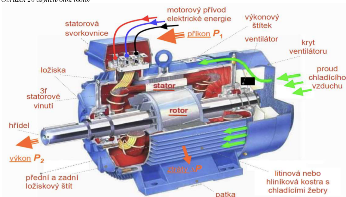
Obrázek 20 asynchronní motor
