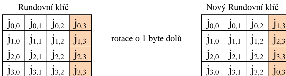
Obrázek 3.8: Operace RotWord
