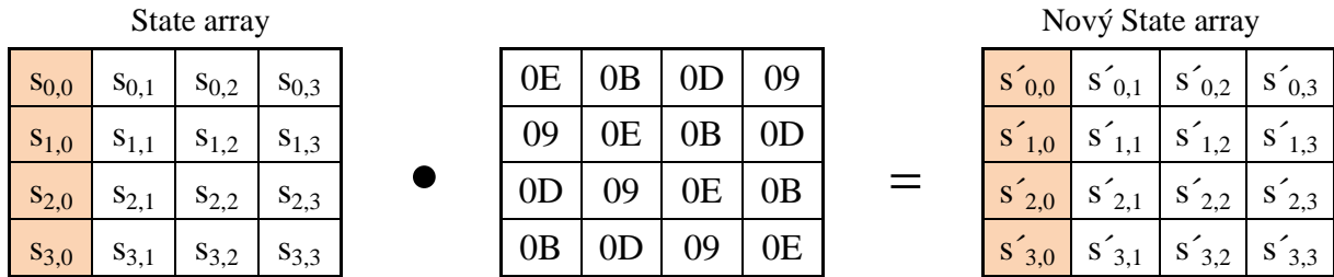
Obrázek 3.6: Operace InvMixColumns
