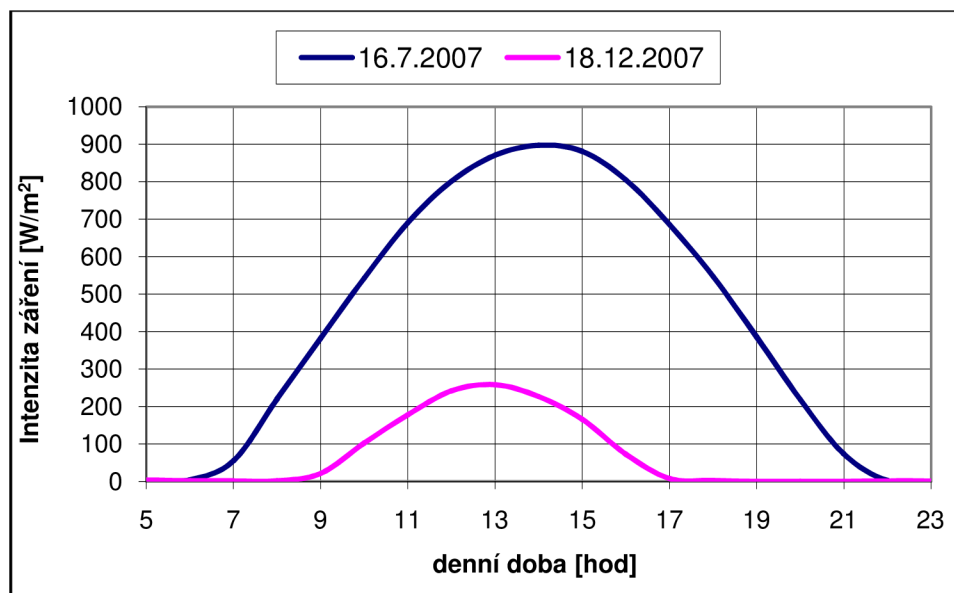
Obr. 4.2 Intenzita globálního záření na vodorovnou plochu slunečního dne v letním období 16. 7. 2007 a v zimním období dne 18. 12. 2007.
