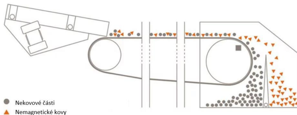
Obr. 20: Odvod frakcí ze separátoru neželezných kovů [41]
