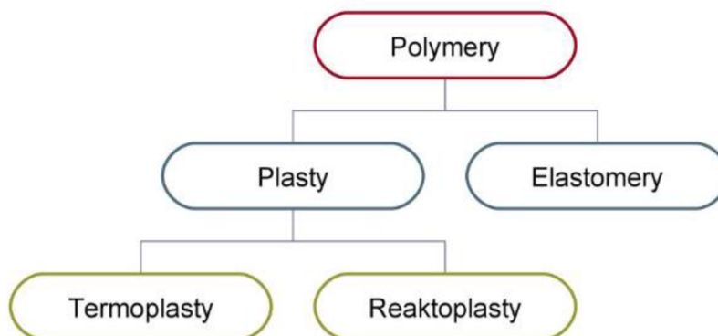
Obr. 2: Rozdělení polymerů [6]
