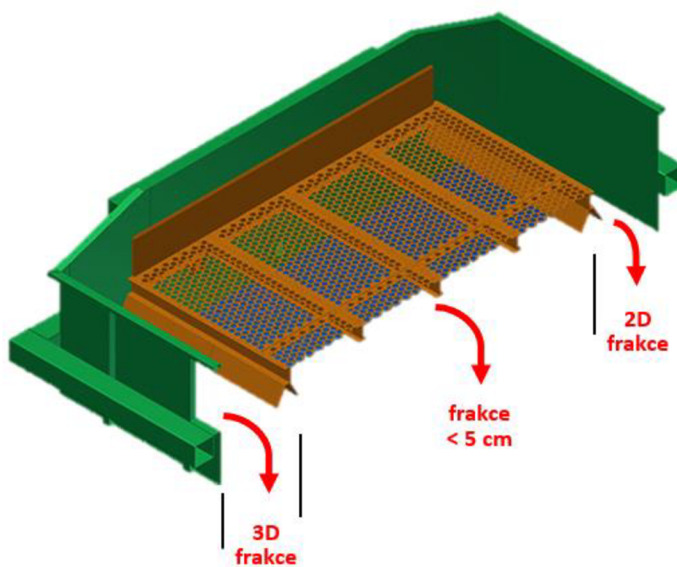
Obr. 19: Odvod frakcí z balistického separátoru [39]
