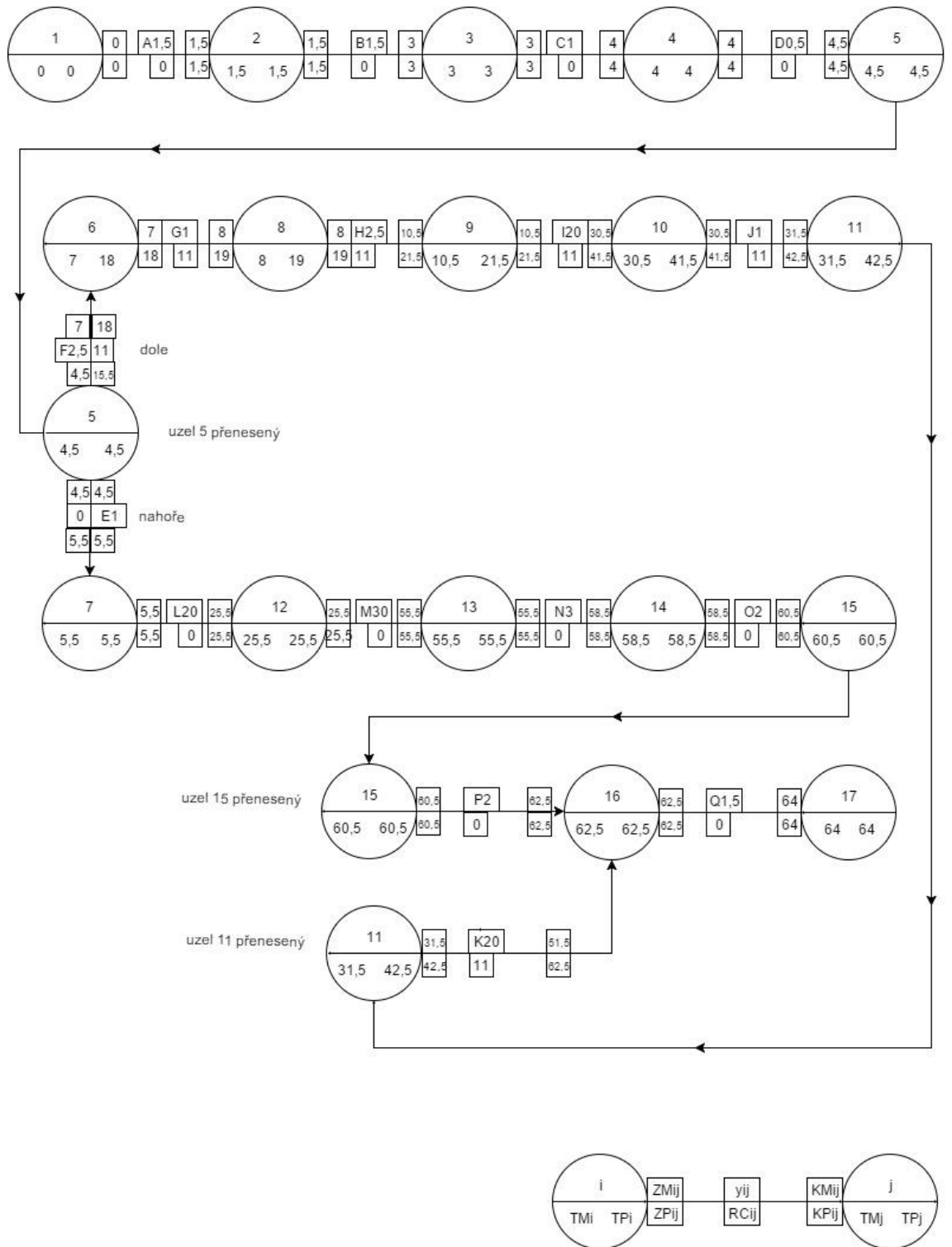
Obrázek č. 7: Síťový graf prodejního procesu (Zdroj: Doskočil, 2011, zpracování: vlastní)
