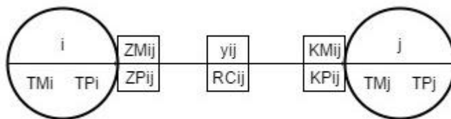
Obrázek č. 2: Popis orientované úsečky síťového grafu (Zdroj: Doskočil, 2011, zpracování: vlastní)
