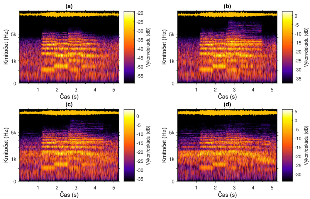
Obr. E.1: Spektrogramy druhé sirény s dopravním ruchem. (a) bez dopravního ruchu; (b) s ruchem dopravní zácpy; (c) s doravním ruchem; (d) s velký dopravním ruchem.
