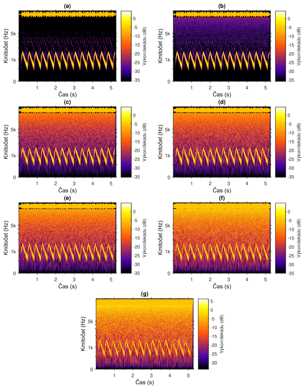
Obr. B.1: Spektrogramy zvuku první sirény s přidáním bílým šumem. (a) bez šumu; (b) bílý šum -20 dBFS; (c) bílý šum -10 dBFS; (d) bílý šum -8 dBFS; (e) bílý šum -6 dBFS; (f) bílý šum -3 dBFS; (g) bílý šum -1 dBFS
