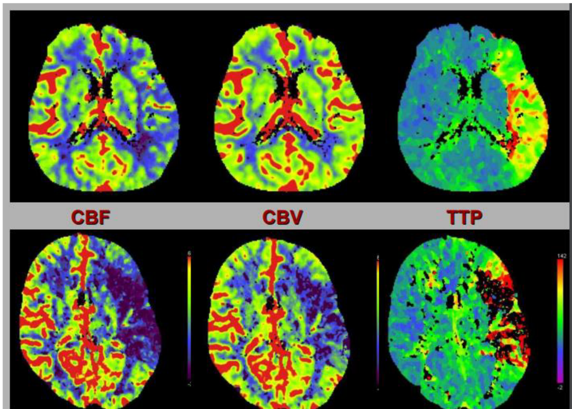
Obrázek 2 Perfuční mapa (Ferda, 2007)
