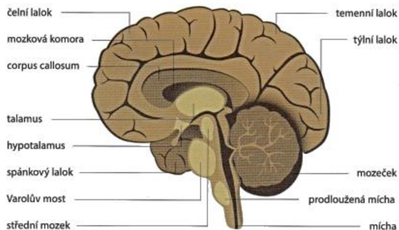
Obrázek 3 Přířez mozem (Wurstová, 2016)
