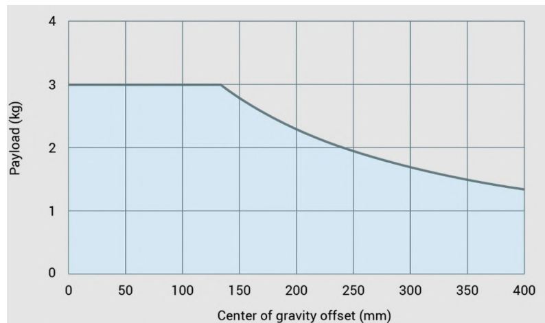
Obrázek 3.2: Graf zatížení [1]
