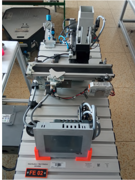
Obrázek 6.1: Distribuční stanice
