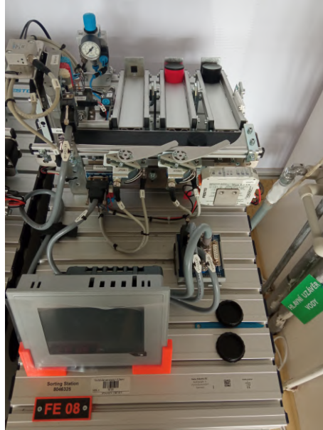
Obrázek 6.5: Třídící stanice
