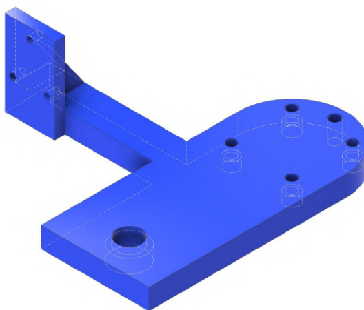
Obrázek 9.1: Model nástroje
