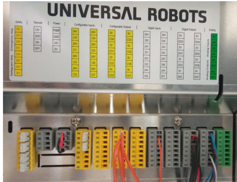
Obrázek 3.4: Konfigurace I/O
