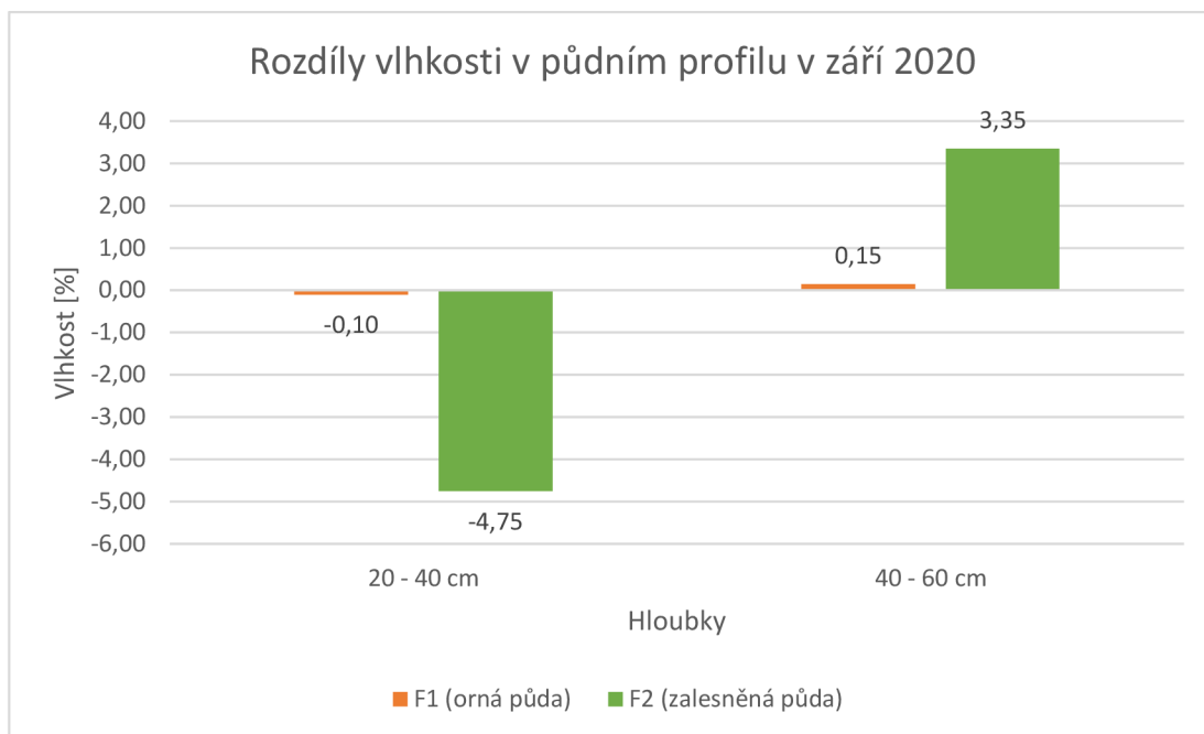
Graf 29: Rozdíly vlhkosti v půdním profilu v září 2020 - Hovorčovice (data: VŮMOP ©2020, graf: autor 2022).
