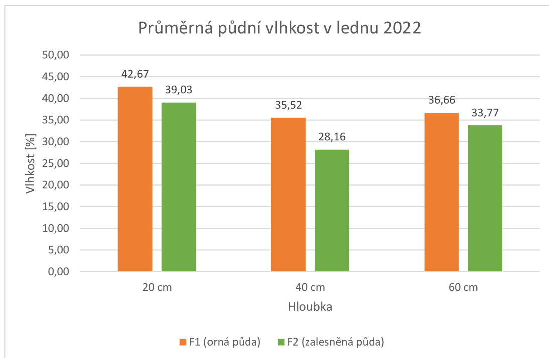
Graf 34: Průměrná půdní vlhkost v lednu 2022 - Hovorčovice (data: VÚMOP ©2020, graf: autor 2022).
