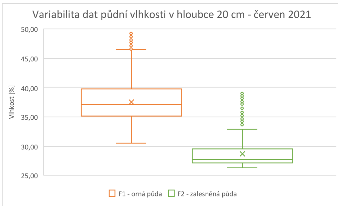
Graf 15: Variabilita dat půdní vlhkosti v hloubce 20 cm - červen 2021 Hovorčovice (data: VŮMOP ©2022, graf: autor 2022).
