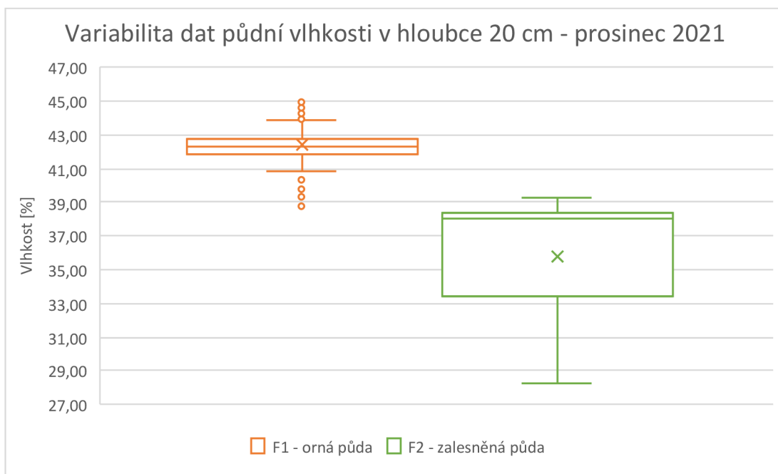
Graf 21: Variabilita dat půdní vlhkosti v hloubce 20 cm - prosinec 2021 Hovorčovice (data: VŮMOP ©2022, graf: autor 2022).
