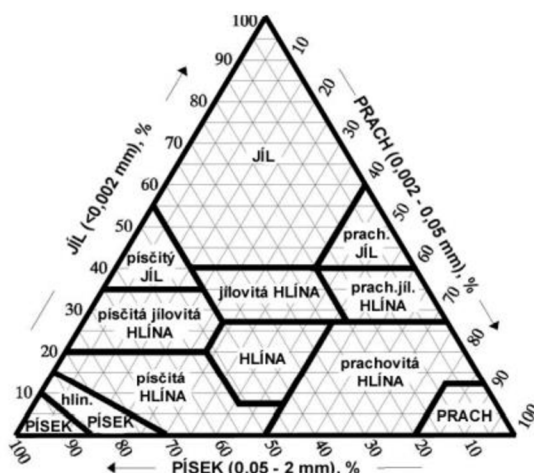
Obrázek 4: Kategorie půdní zrnitosti podle systému USDA (Pavluš 2018).
