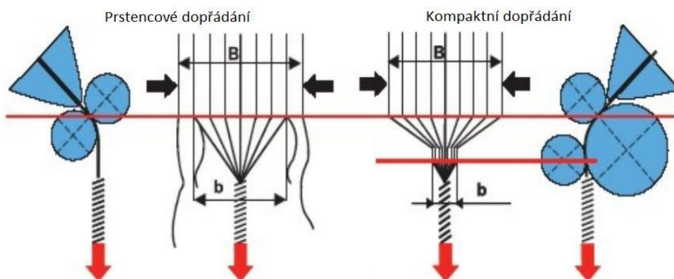
Obr 3 Prádní trojúhelník (vlevo klasické prstencové dopřádání, vpravo kompaktní dopřádání)
