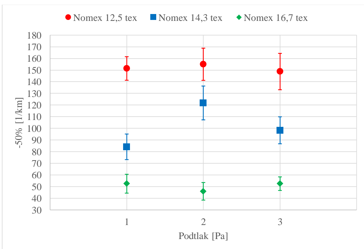
Obr. 11 Graf – slabá místa -50% příze Nomex
