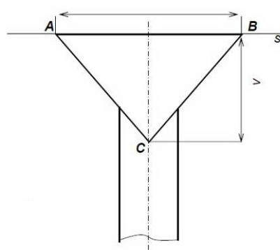
Obr.4 Schéma prádního trojúhelníku
