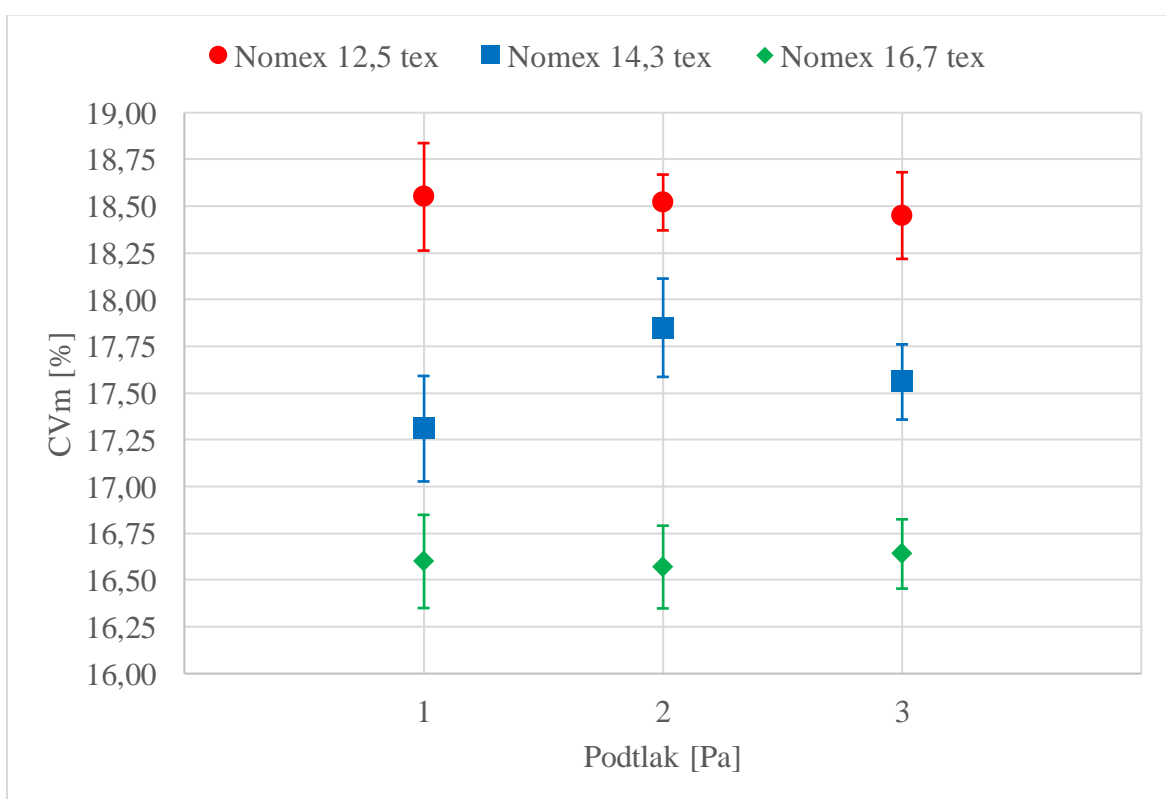
Obr. 9 Graf – kvadratická nestejnomyčnost CVm příze Nomex
