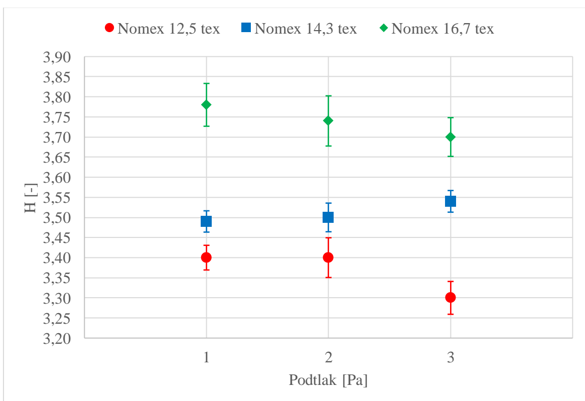
Obr. 17 Graf – chlupatost H přize Nomex
