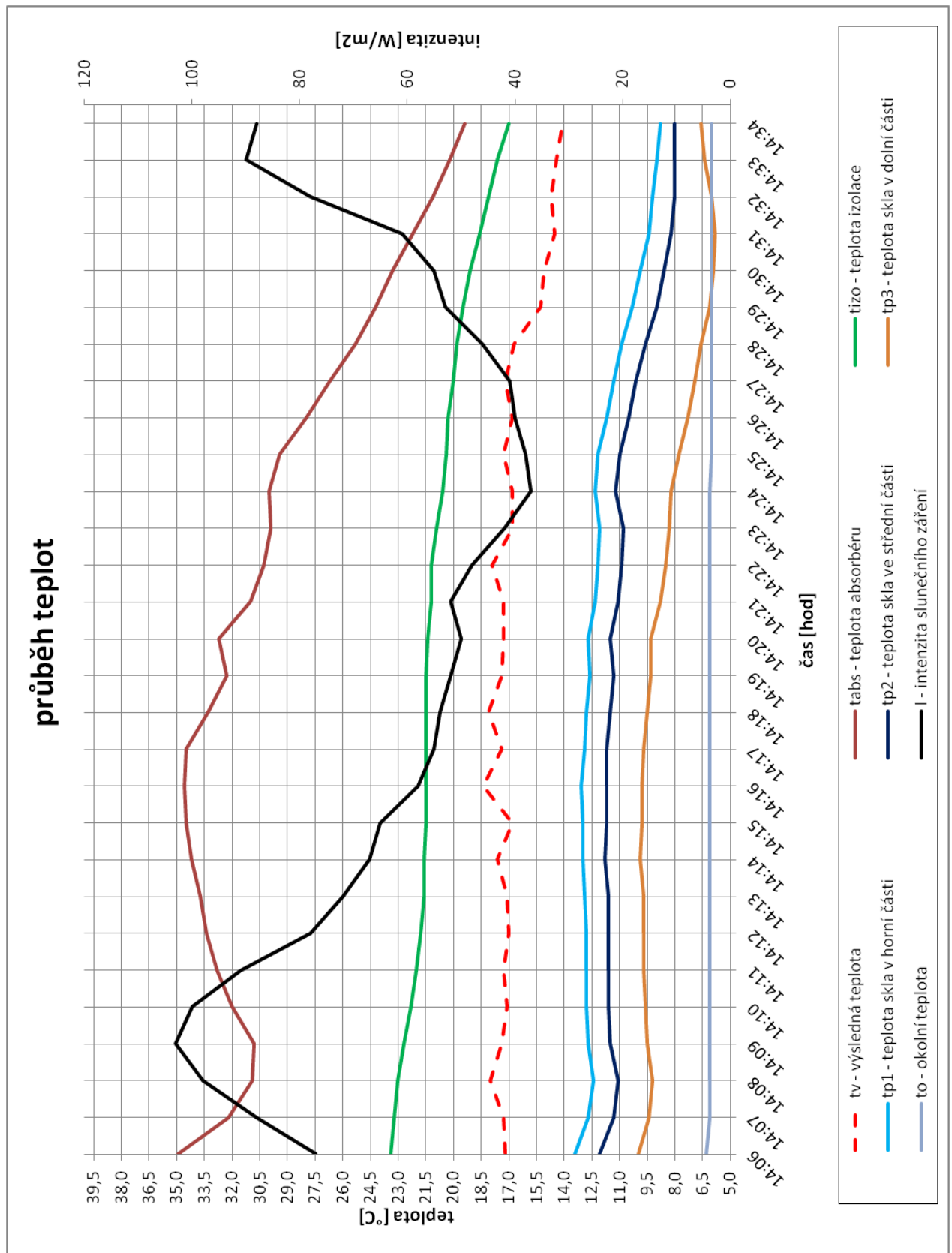
Graf 7: průběh teplot a intenzity slunečního záření - II. etapa 2. měření
