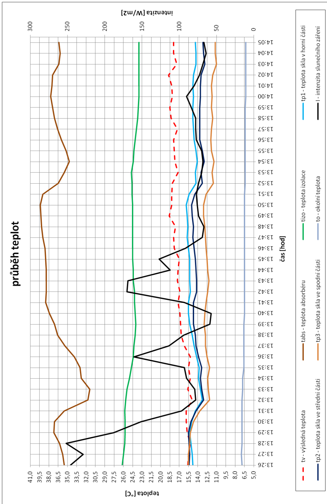
Graf 5: průběh teplot a intenzity slunečního záření - I. etapa 2. měření
