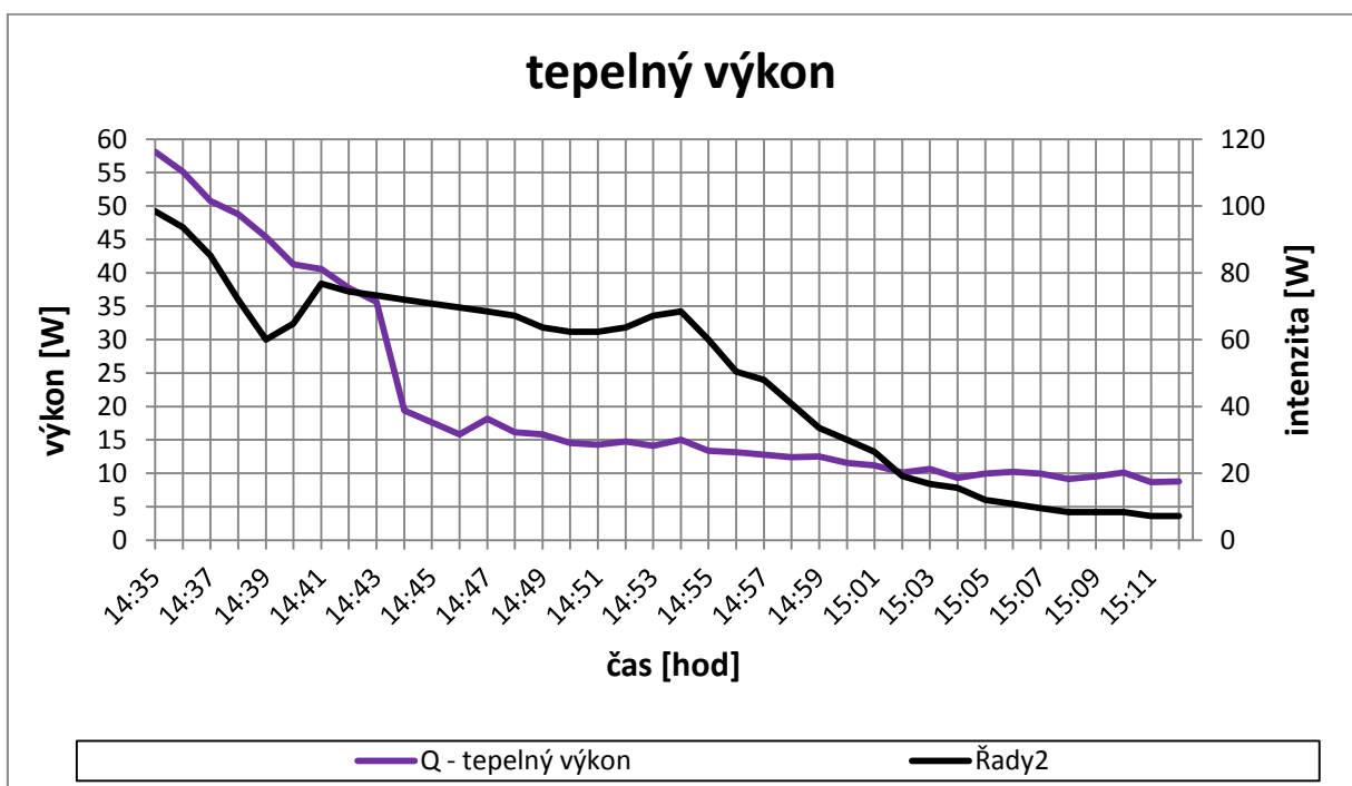
Graf 10: průběh tepelného výkonu 2. měření - III. etapa
