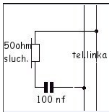
Obr. 3.5: Znázorněné zapojení odposlechu telefonní linky se sluchátkem.
