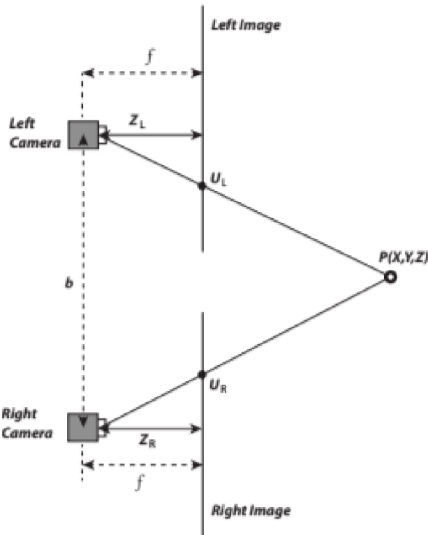
Obrázek 13 Geometrie hloubky ve stereokamerách [16]
