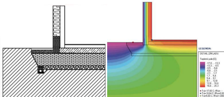
Obrázek 24 Konstrukční detail – klasicky vyztužená deska na podsypu z Liaporu (vlevo), simulace teplotních polí (vpravo) [46]
