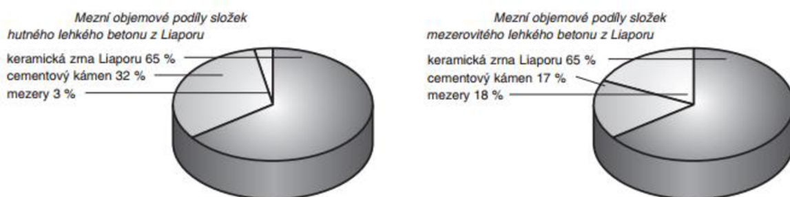
Obrázek 18 Mezní podíly hutného a mezerovitého lehkého betonu [5]
