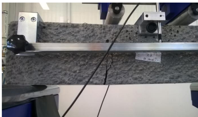
Obrázek 36 Poloha makrotrhliny
