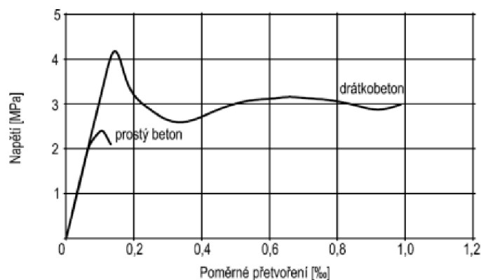
Obrázek 9 Pracovní diagram drátkobetonu v tahu [1]
