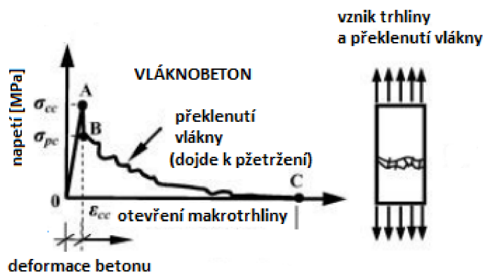
Obrázek 10 Beton vyšších tříd – přetržení vlákna [11]
