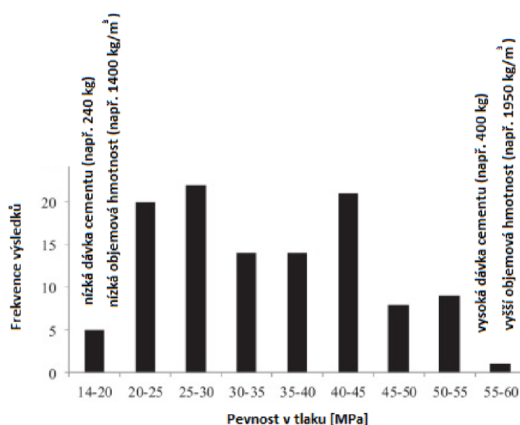
Obrázek 21 Frekvence dosažených výsledků pevností v tlaku [36]
