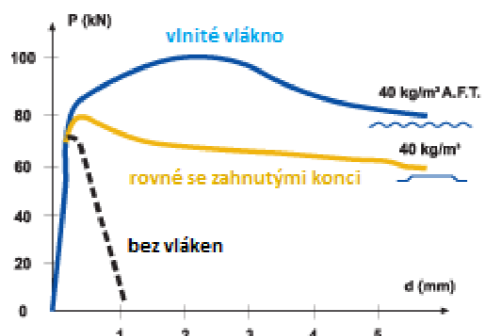
Obrázek 6 Srovnání pracovních diagramů dle tvaru vláken [6]
