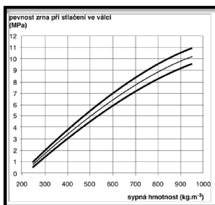
Obrázek 2 Průběh pevnosti v tlaku v závislosti na sypané hmotnosti [2]
