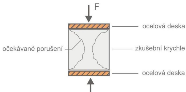
Obrázek 30 Schéma zkoušky pevnosti v tlaku [17]
