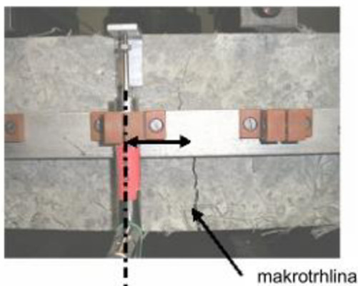
Obrázek 33 Poloha makrotrhliny [30]
