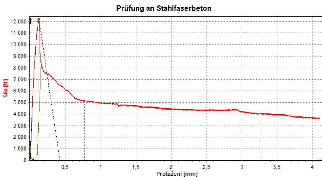
Graf 8 Výkonový diagram na trávci č. 2 700×150×150
