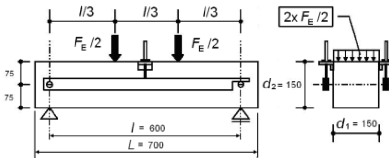
Obrázek 32 Uspořádání zkoušky [30]
