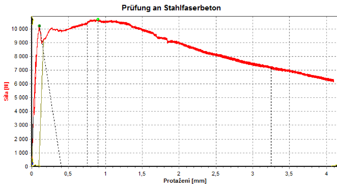
Graf 7 Výkonový diagram na trávci č. 1 700×150×150
