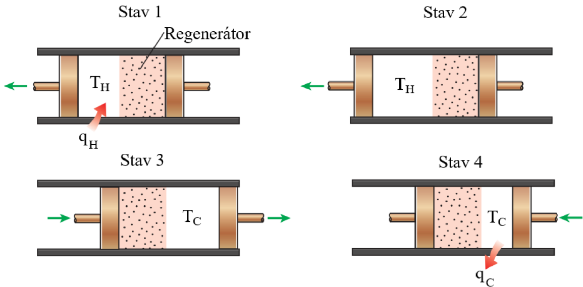
Obr. 5.6: Schéma teoretického provedení Stirlingova cyklu, upraveno dle [24].
