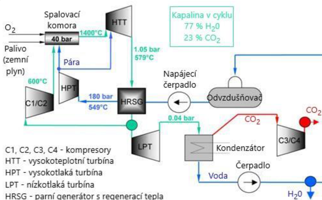
Obr. 5.9: Schéma Graského cyklu, upraveno dle [40].
