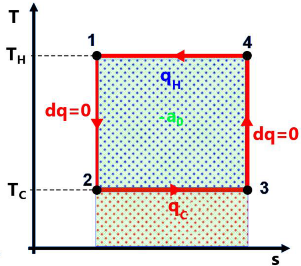
Obr. 1.5: T - s diagram obráceného Carnotova cyklu, upraveno dle [5].
