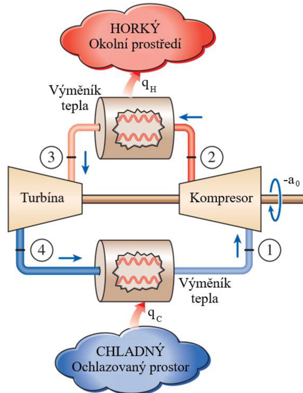
Obr. 4.12: Schéma Bell Colemanova cyklu, upraveno dle [29].
