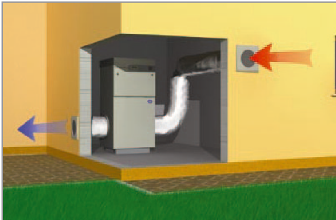
Obr. 1.6 Vnitřní provedení
