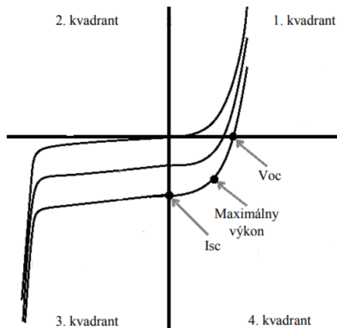
Obrázok 3-8 VA-charakteristika fotodiódy [13]
