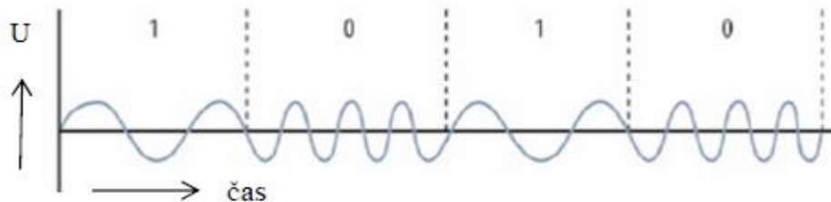
Obrázok 4-3 FSK modulácia [20]
