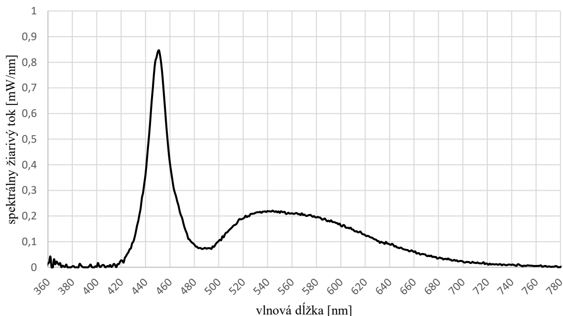
Obrázok 6-5 Spektrum zostrojeného svetidla
