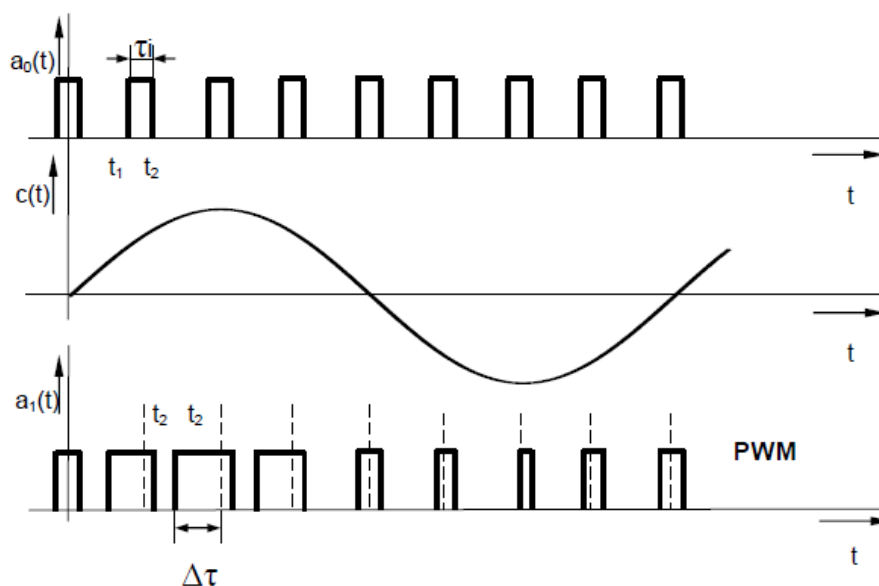
Obrázok 4-5 PWM modulácia [20]
