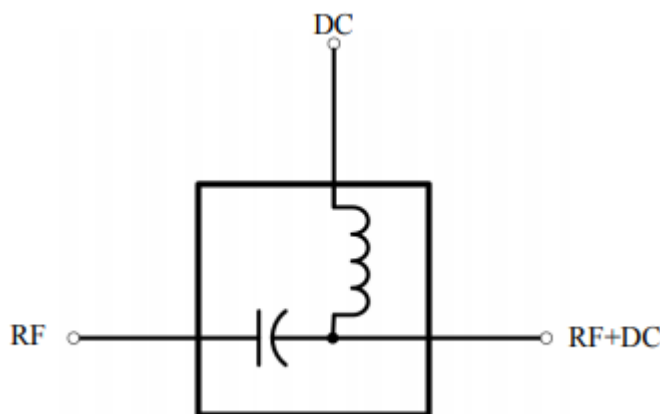
Obrázok 3-4 Obvod Bias-T [13]
