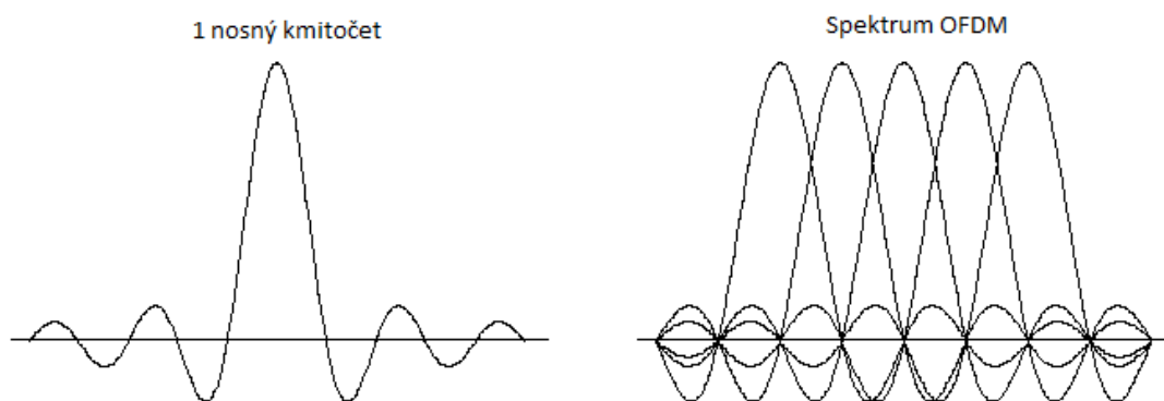
Obrázok 4-4 OFDM modulácia [22]
