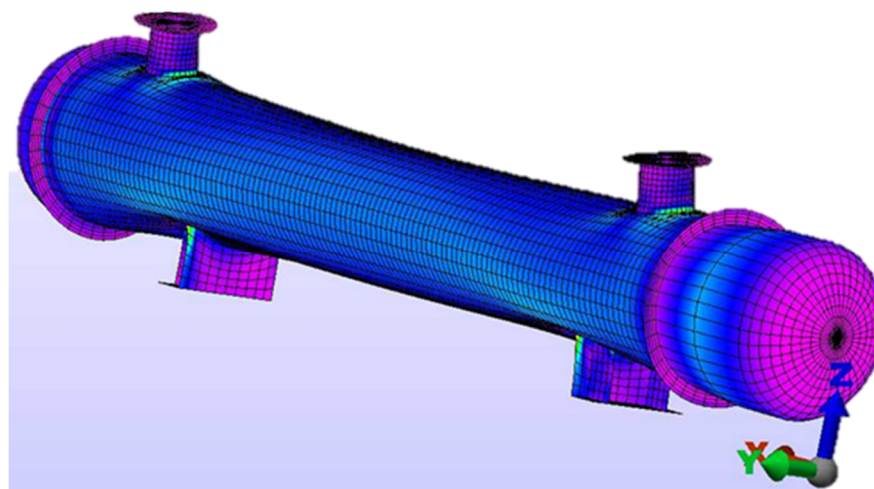
Obr 4.1.1 Síť prvků na výměníku tepla [12]
