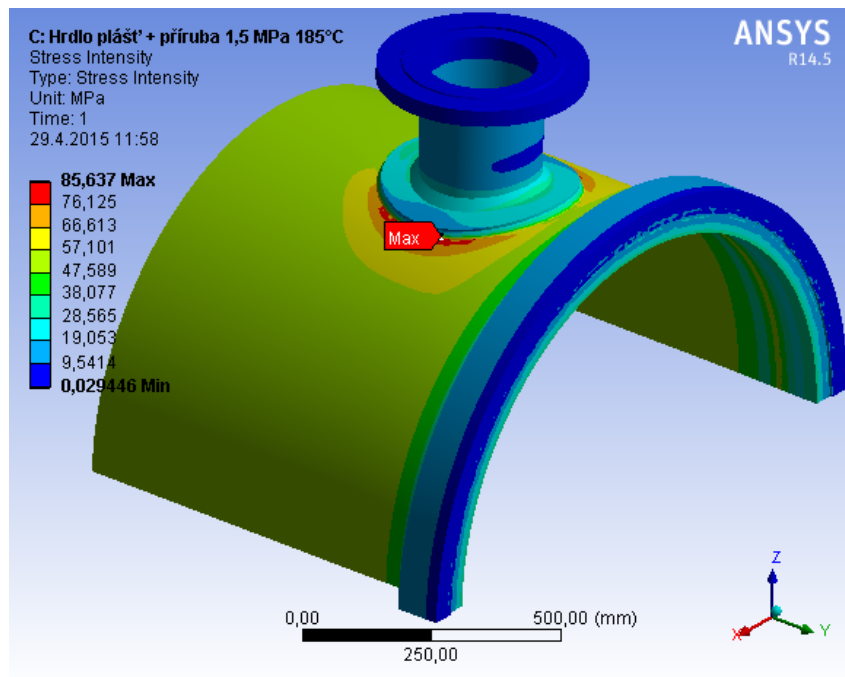
Obr 4.1.8 Intenzita napětí- VP
