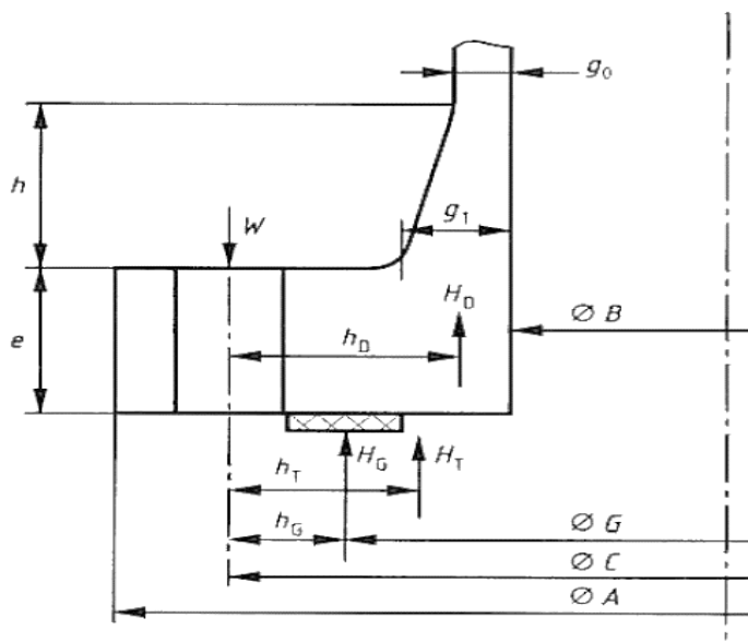
Obr 3.6.1 Schéma přírubby [8]
