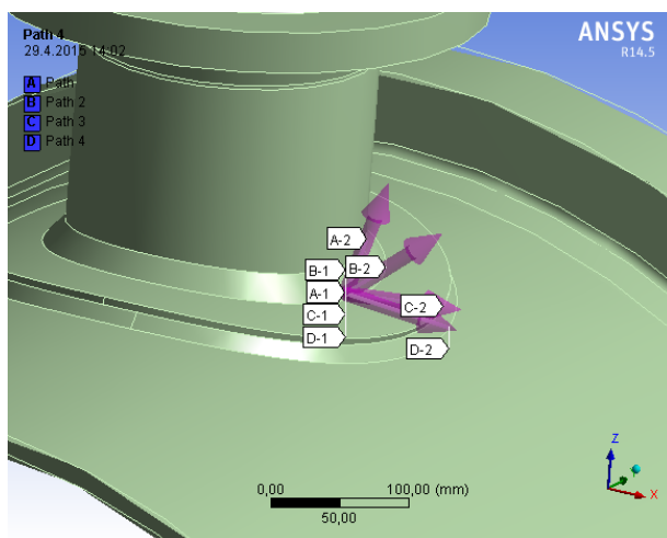
Obr. 4.1.12 Linearizační přímký- VP
