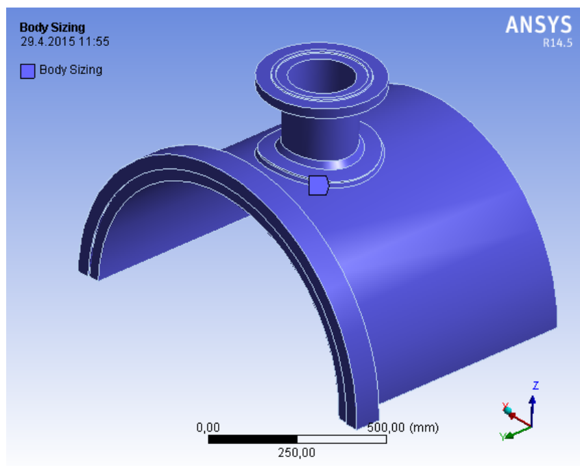
Obr 4.1.3 Modifikace sítě
