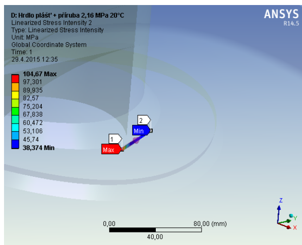
Obr. 4.1.17 Průběh napětí B1/B2- ZP
