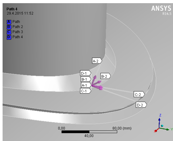
Obr. 4.1.13.1 Linearizační přímký- ZP
