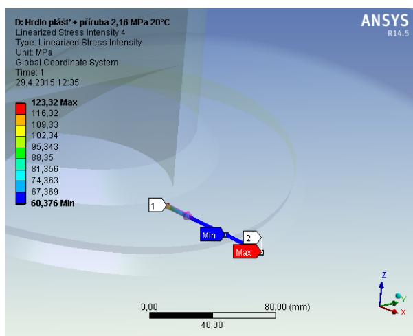
Obr. 4.1.19 Průběh napětí C1/C2- ZP
