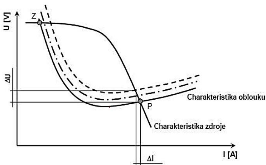
Obr. 10 Spojení charakteristik [14]
