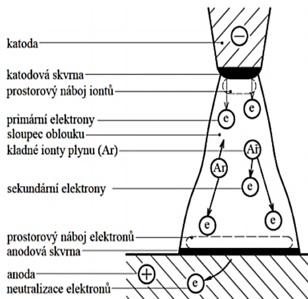
Obr. 8 Elektrický oblouk [1]
