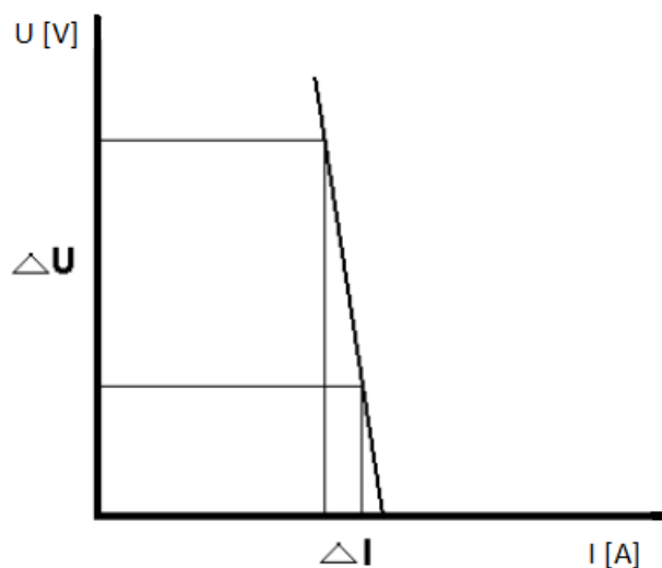
Obr. 9 Strmá charakteristika [13]
