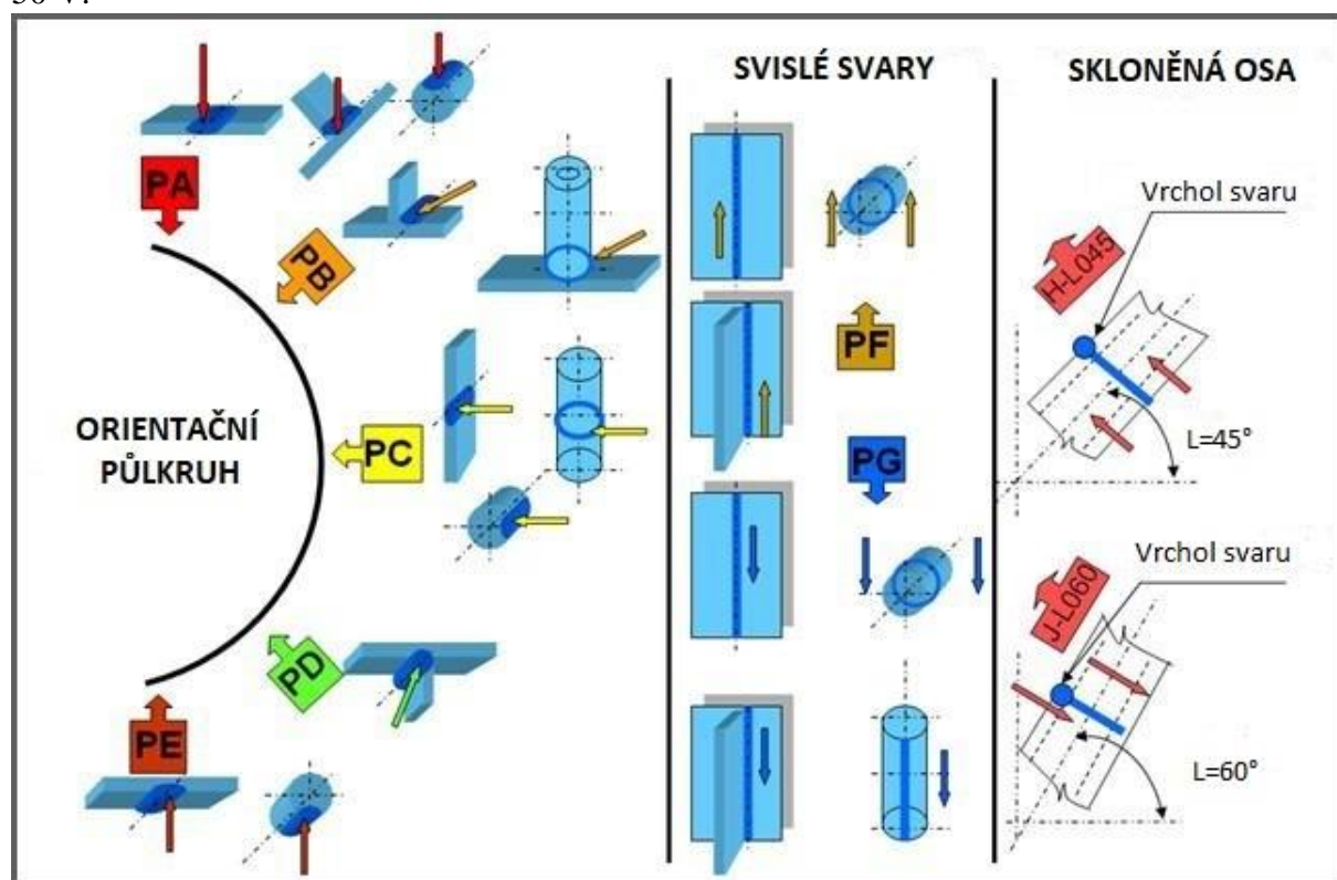
Obr. 7 Polohy svařování [9]
