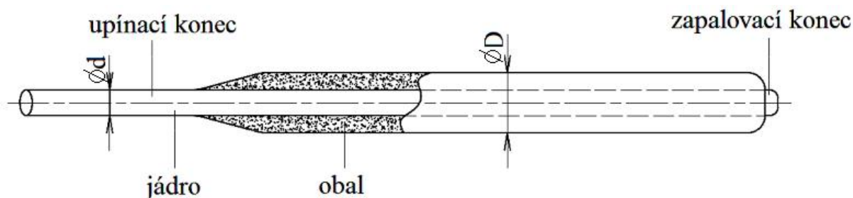
Obr. 11 Obalovaná elektroda [13]
