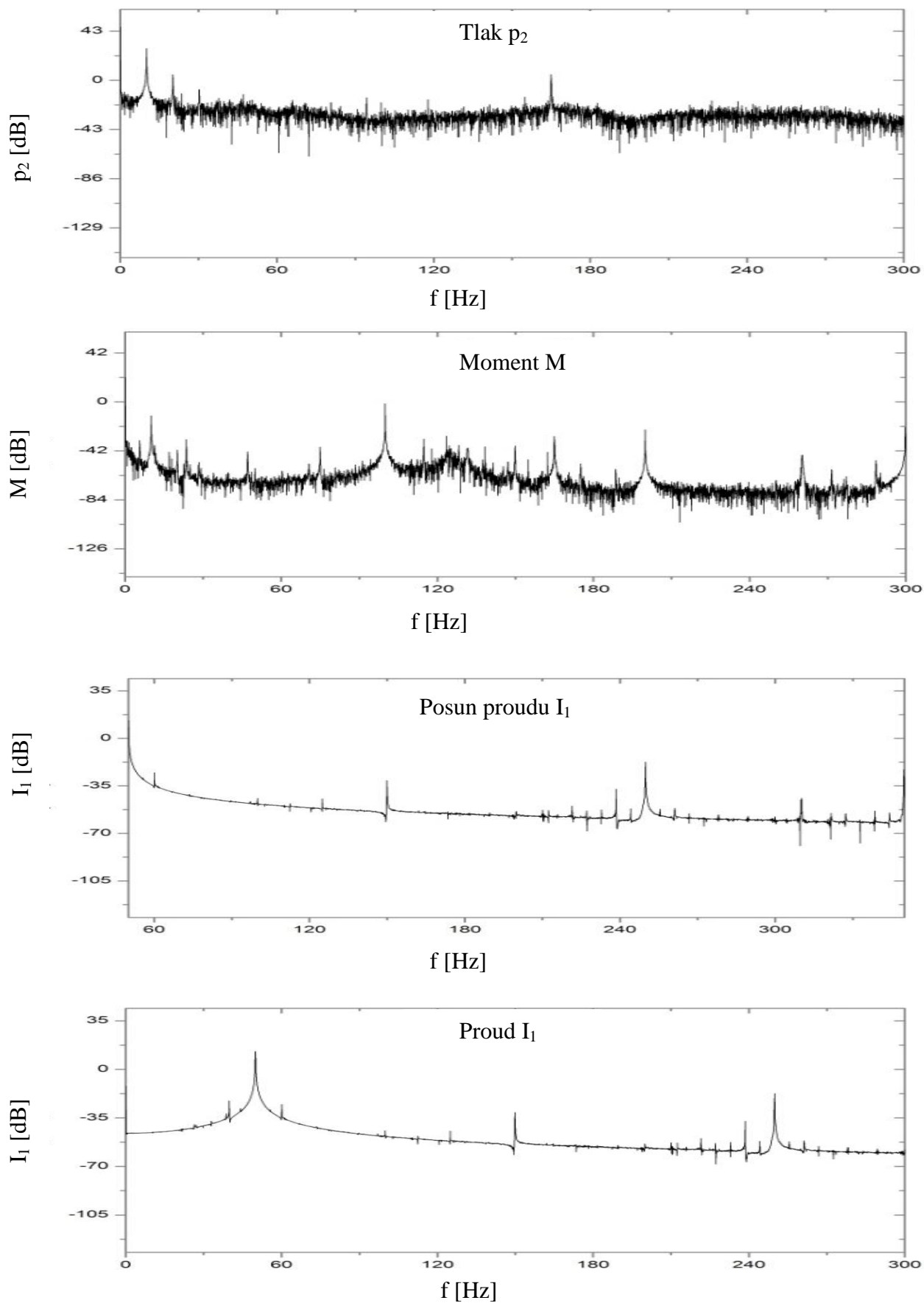
Obrázek 26: Grafy závislosti útlumu na frekvenci pro jednotlivé veličiny, f=10\text{Hz} , Q=10l
