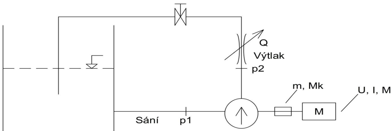
Obrázek 14: Schéma zapojení pracoviště
