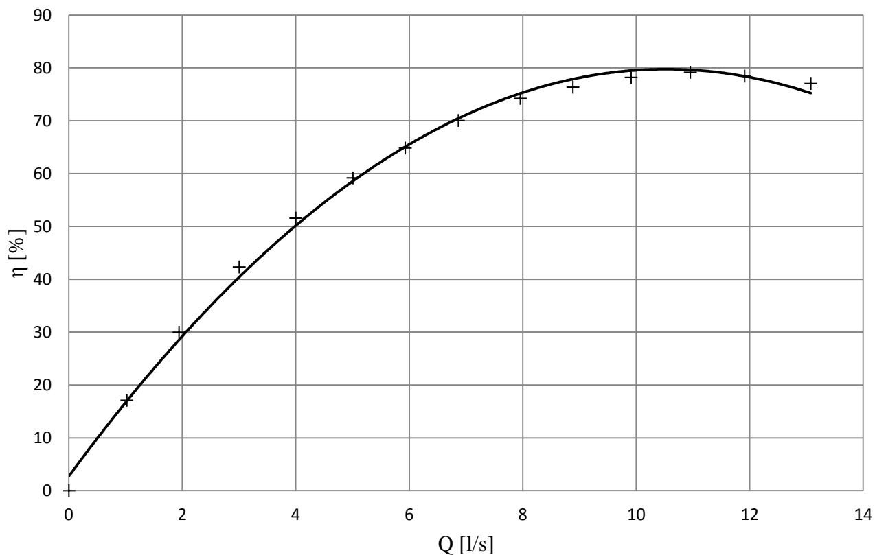
Obrázek 19: Graf závislosti účinnosti čerpadla na průtoku
