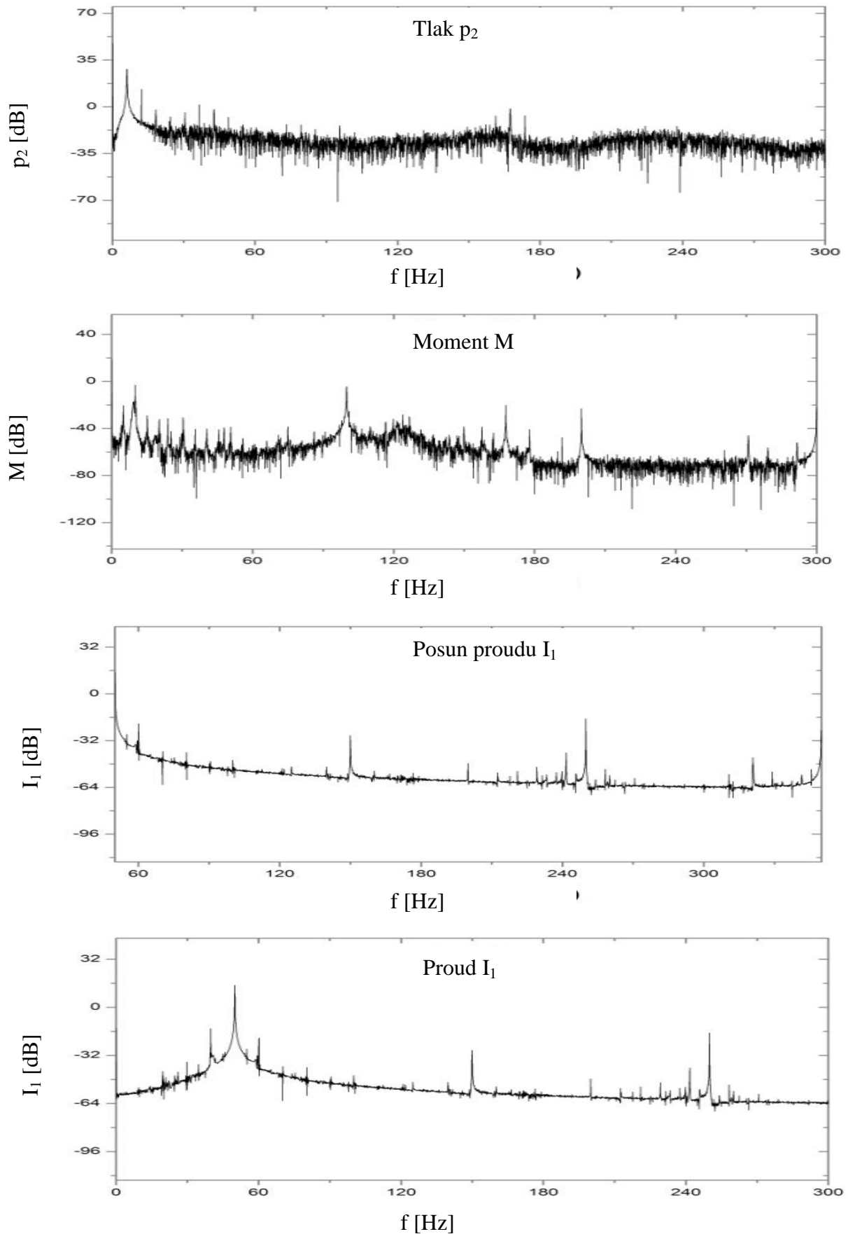
Obrázek 30: Grafy závislosti útlumu na frekvenci pro jednotlivé veličiny, f=10\text{Hz} , Q=61
