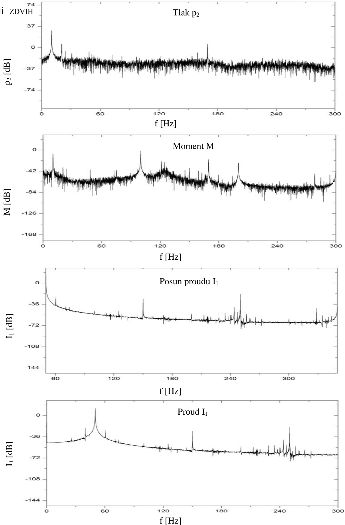
Obrázek 23: Grafy závislosti útlumu na frekvenci pro jednotlivé veličiny, f=10\text{Hz} , Q=31
