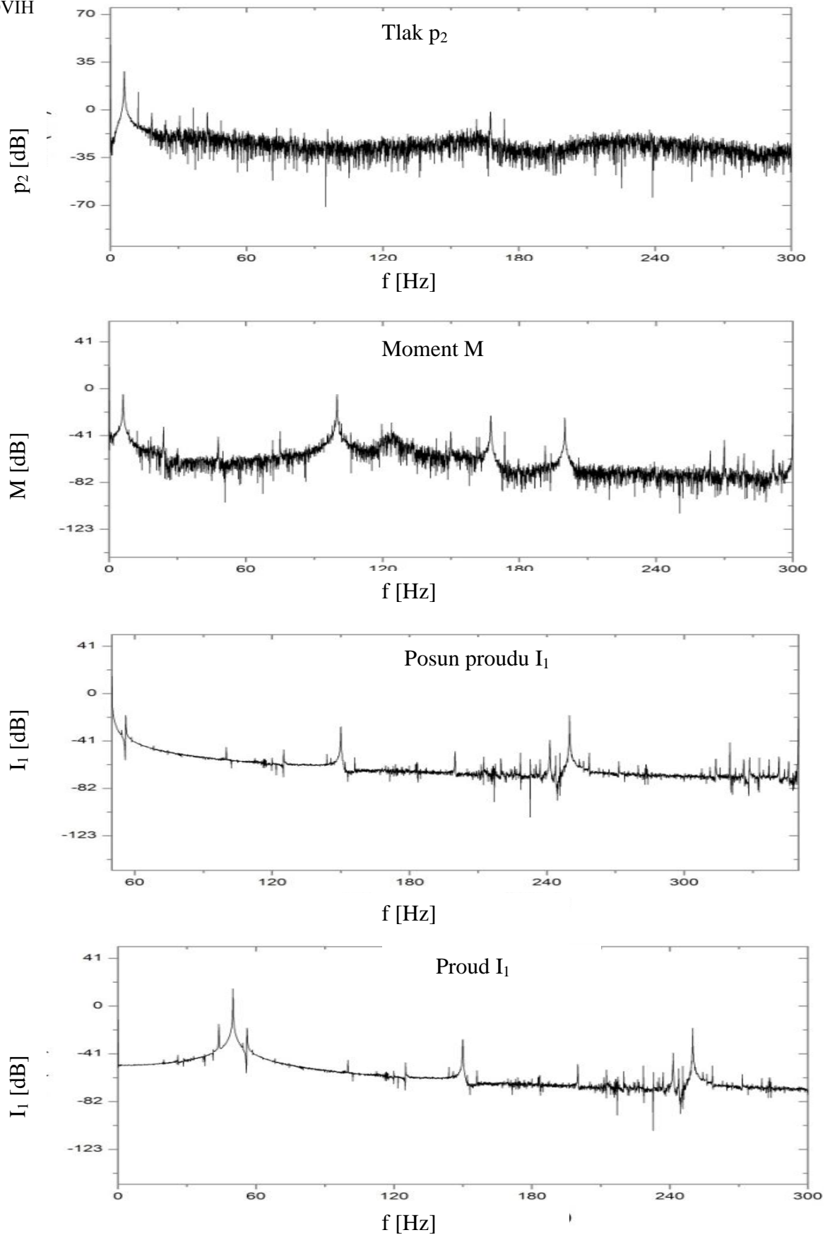
Obrázek 28: Grafy závislosti útlumu na frekvenci pro jednotlivé veličiny, f=6\text{Hz} , Q=61
