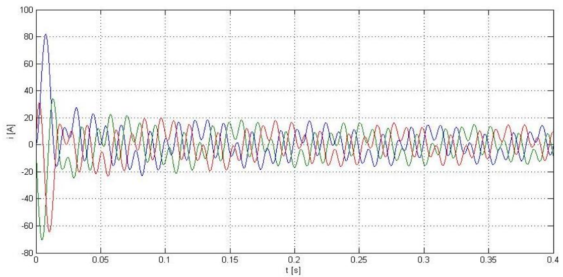
Obrázek 35: Grafy závislosti proudu na čase pro f=10\text{Hz} , Q=10\text{l} , motor 2
