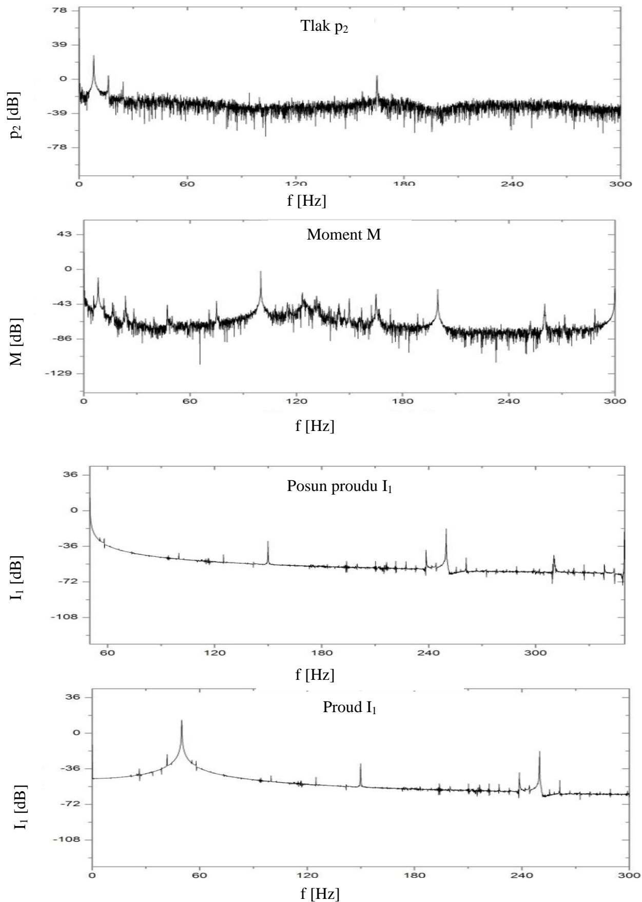
Obrázek 25: Grafy závislosti útlumu na frekvenci pro jednotlivé veličiny, f=8\text{Hz} , Q=10l
