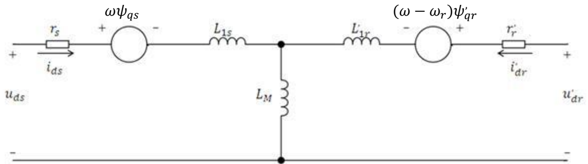
Obrázek 6: Obvodový model vztažený pro osu d [4]
