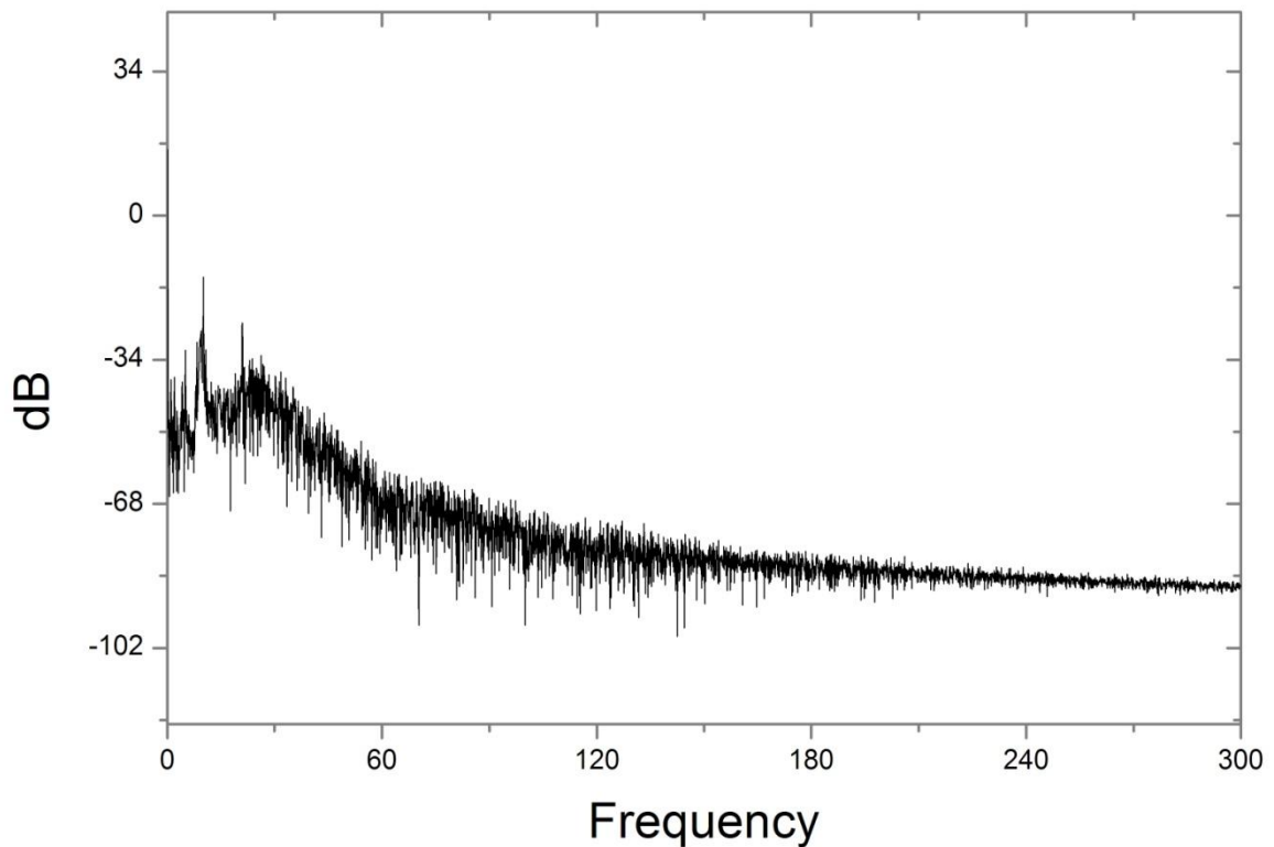
Obrázek 33: Fourierova transformace horní obálky f=10\text{Hz} , Q=6 l, celý časový rozsah
