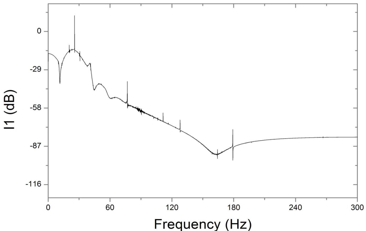
Obrázek 36: FFT proudu I_1 při buzení momentem
