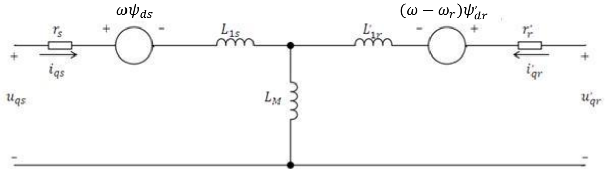
Obrázek 5: Obvodový model vztažený na osu q [4]
