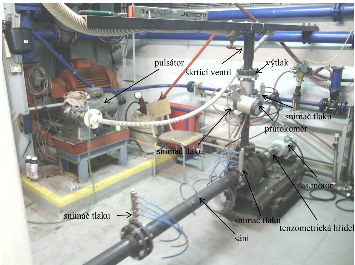
Obrázek 15: Pohled na zapojené pracoviště
