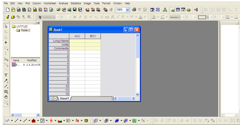
Obrázek 3: Prostředí OriginPro
