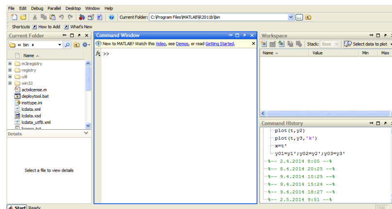
Obrázek 4: Prostředí Matlab
