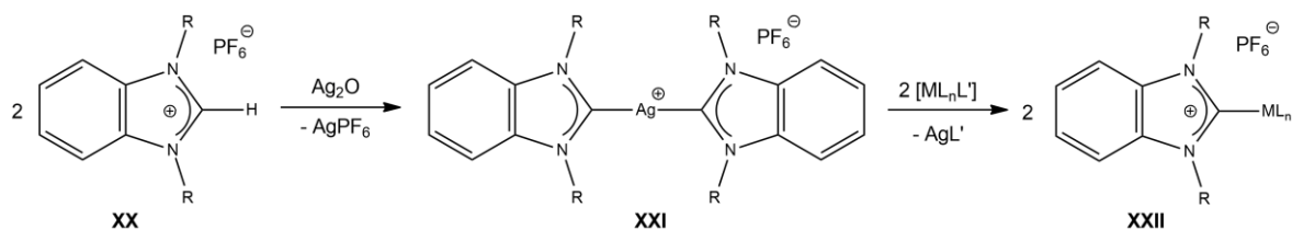
Obrázek 9: Příprava NHC komplexů metodou s \text{Ag}_2\text{O} [9]
