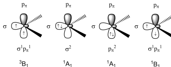
Obrázek 5: Možné elektronové konfigurace karbenů [14]
