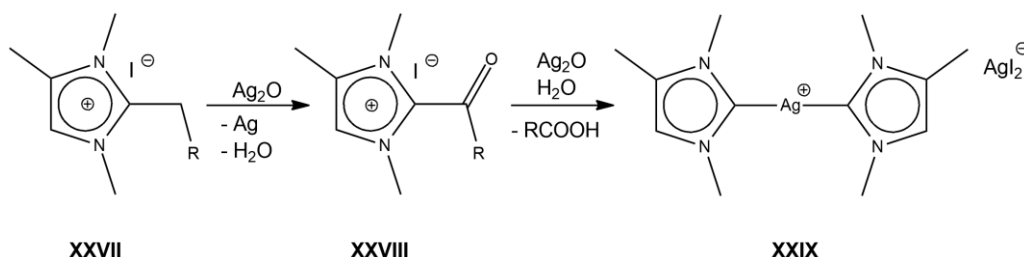
Obrázek 12: Příklad oxidace chránící skupiny oxidem stříbrným [18]
