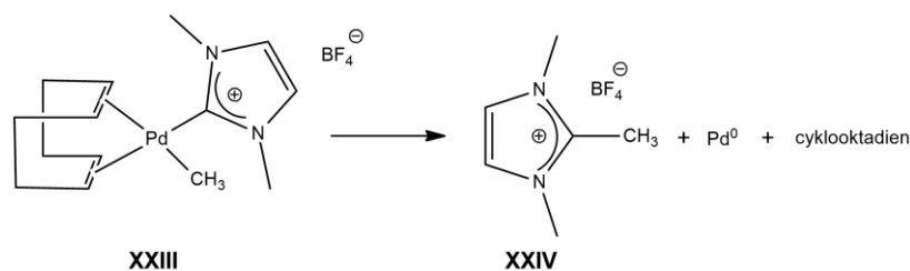
Obrázek 10: Rozklad palladnatého NHC komplexu reductivní eliminací [9]
