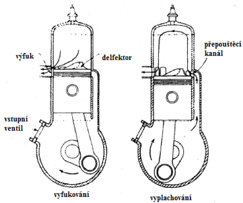
Obr. 2 Cyklus dvoudobého motoru [2]
