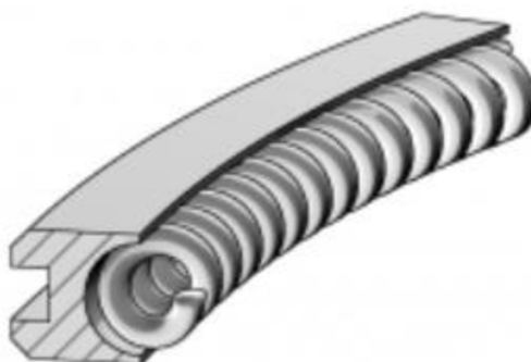
Obr. 18 Dvoudílný stírací kroužek se zkosením [11]
