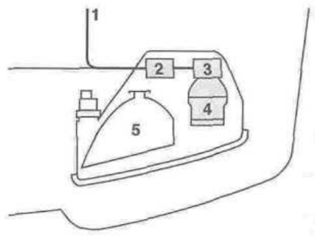
OBR.30:ULOŽENÍ SYSTÉMU LITRONIC [29]
