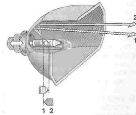
OBR.28:UKÁZKA NASTAVOVÁNÍ TLUMENÝCH A DÁLKOVÝCH SVĚTEL REFLEXNÍ[29]
