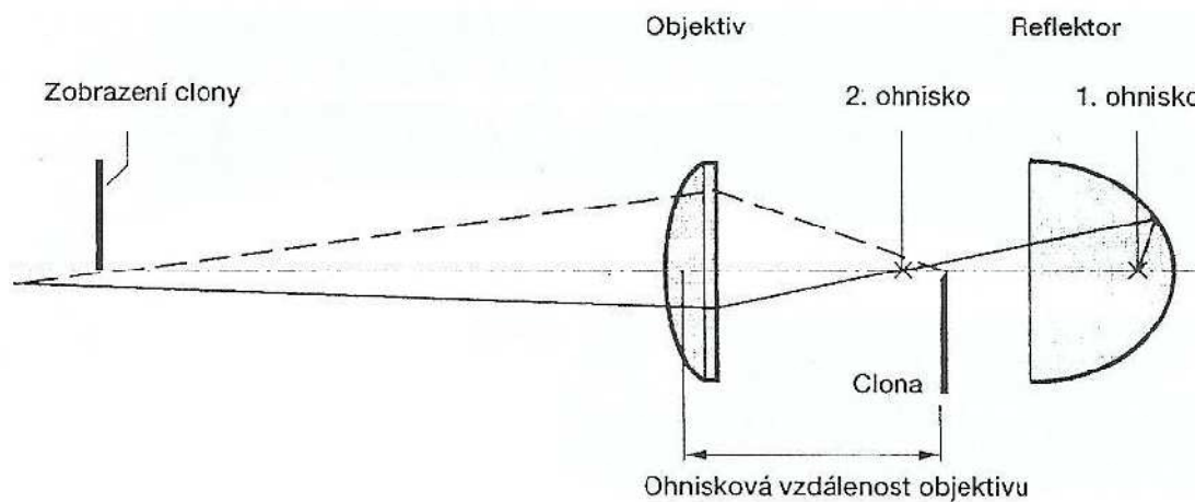
OBR. 21:SCHEMA PRINCIPU PROJEKČNÍCH SYSTÉMŮ[14]
