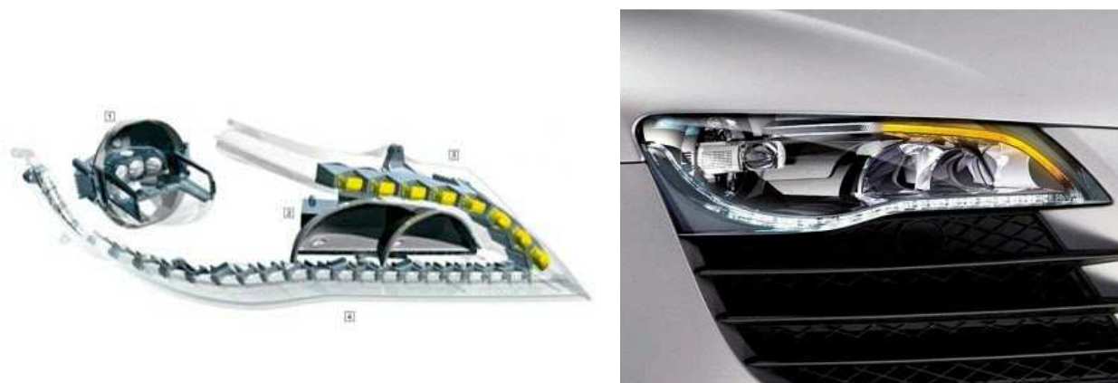
OBR. 15: KONCEPT POUŽITÍ LED DIOD SCHEMA (VLEVO), REÁLNÝ SVĚTLOMET (VLEVO) [11]
