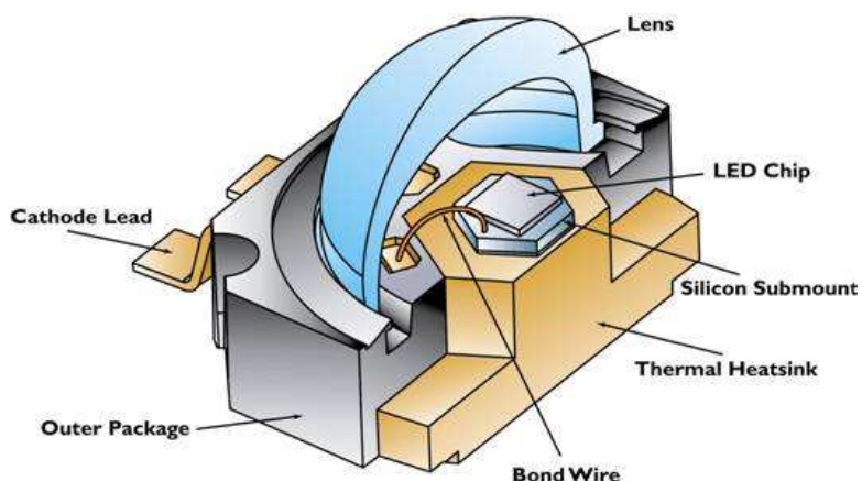
OBR. 17: LUXEON K2 LED DIODA V ŘEZU [32]
