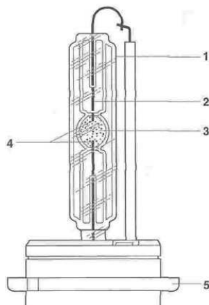
OBR.9: SCHÉMA XENONOVÉ VÝBOJKY D2S [8]
