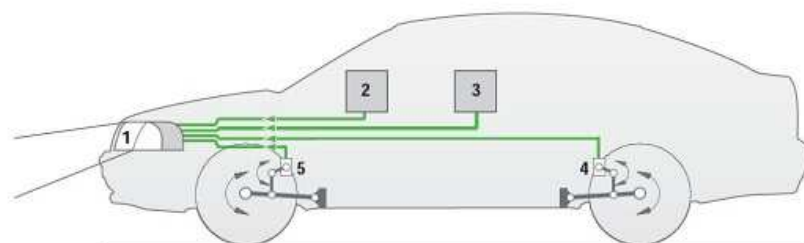
OBR.14: ROZPIS POZICÍ SENZORŮ REGULACI SKOLNU SVĚTLOMETŮ [3]
