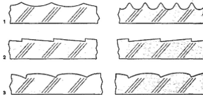
OBR. 18:TVARY ELEMENTŮ NA KRYCÍM SKLE SVĚTLOMETU[7]
