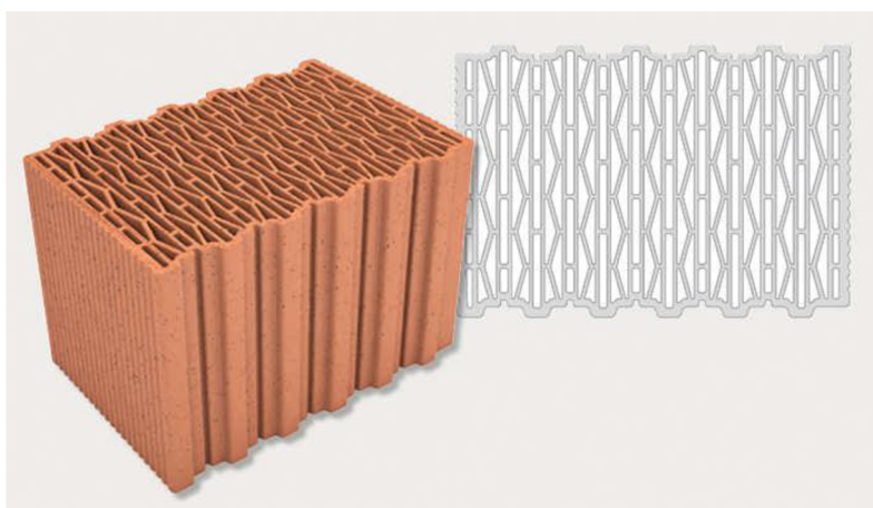
Obrázek 23: THERMOPOR SL [30]
