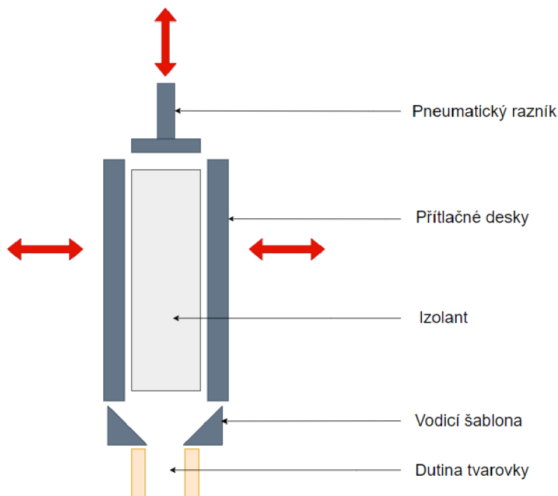
Obrázek 29: Schéma plnění tvarovek pomocí přitlačných desek.
