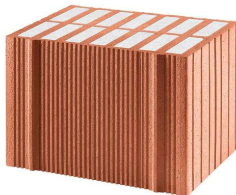
Obrázek 15: POROTON S8 [28]
