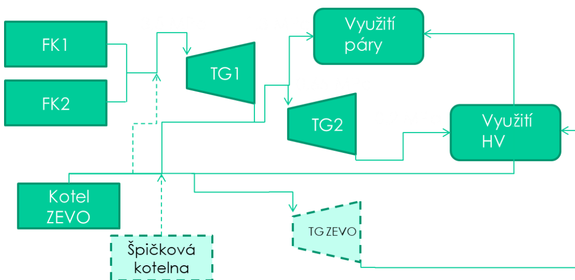
Obr. 45: Blokové schéma vstupující do modelu synergie zařízení EVO s dalším tepelným zdrojem
