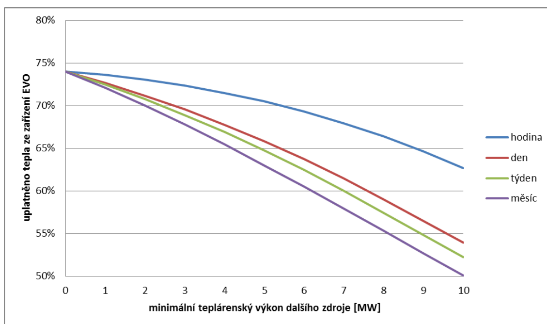
Obr. 34: Závislost množství uplatněného tepla z jednotky EVO na minimálním výkonu dalšího zdroje tepla při různých minimálních dobách jeho odstávků
