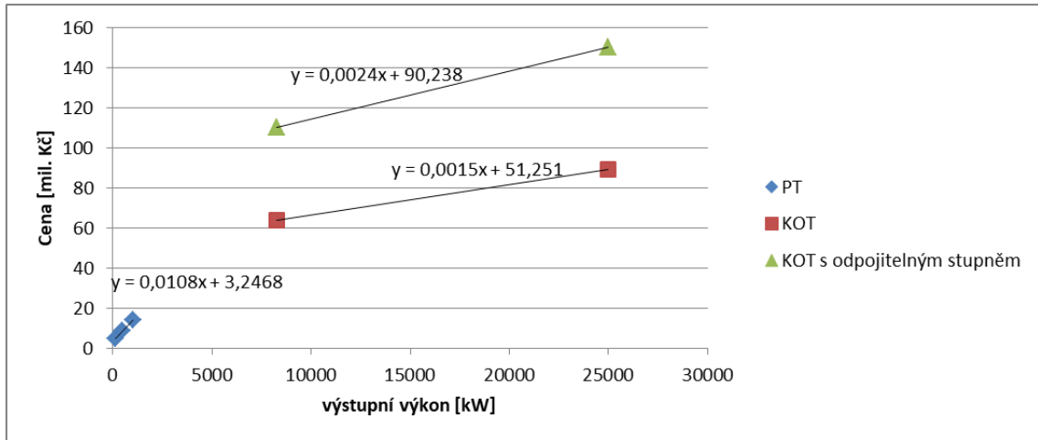
Obr. 35: Investiční náklady parních turbín
