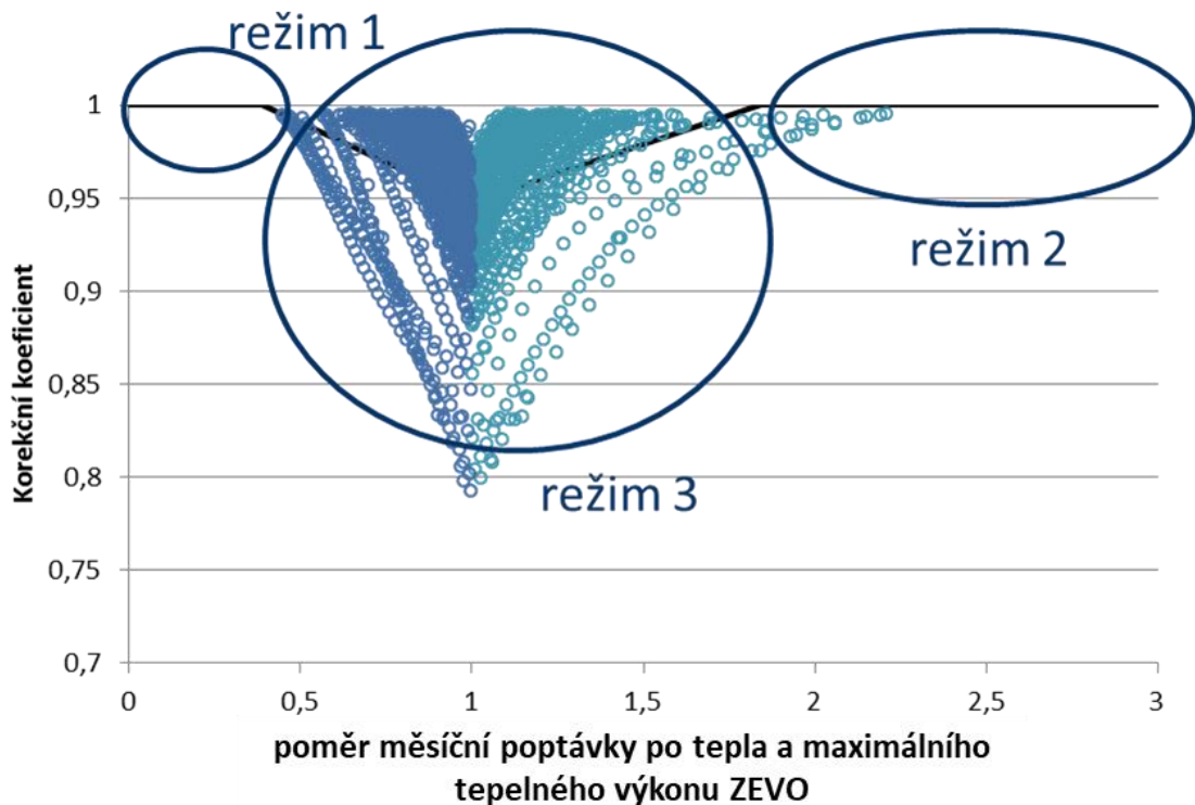
Obr. 32: Závislost korekčního koeficientu na poměru měsíčního požadavku v síti CZT a maximální teoretické měsíční dodávky ze zařízení EVO
