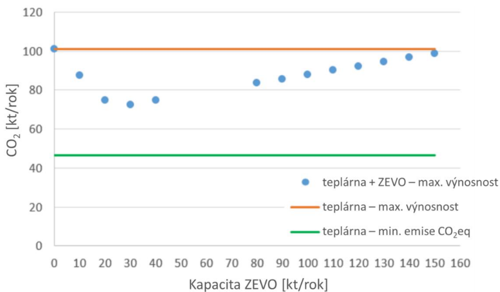
Obr. 50 Emise \text{CO}_2 pro různé režimy provozu
