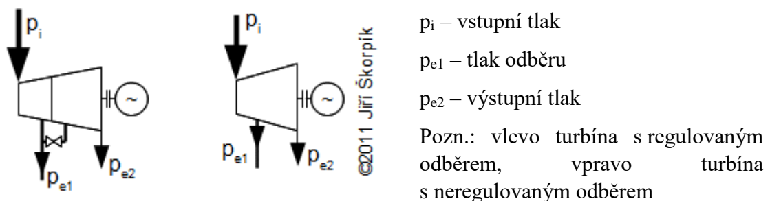
Obr. 13 Zapojení kondenzační odběrové turbíny [59]
