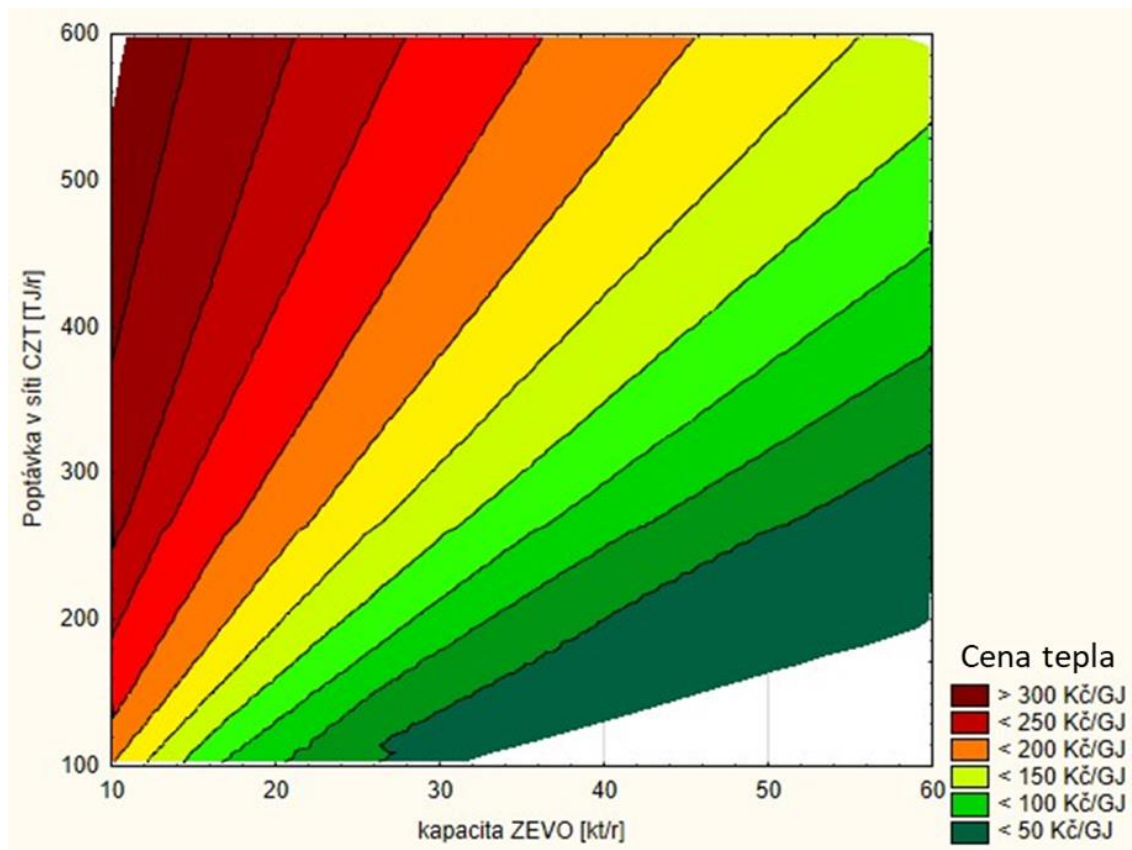
Obr. 41 Závislost nákladů na provoz plynové kotelny vztahených na dodané teplo
