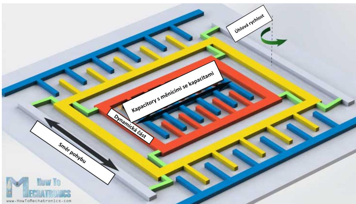
Obrázek 9 MEMS gyroskop [10]
