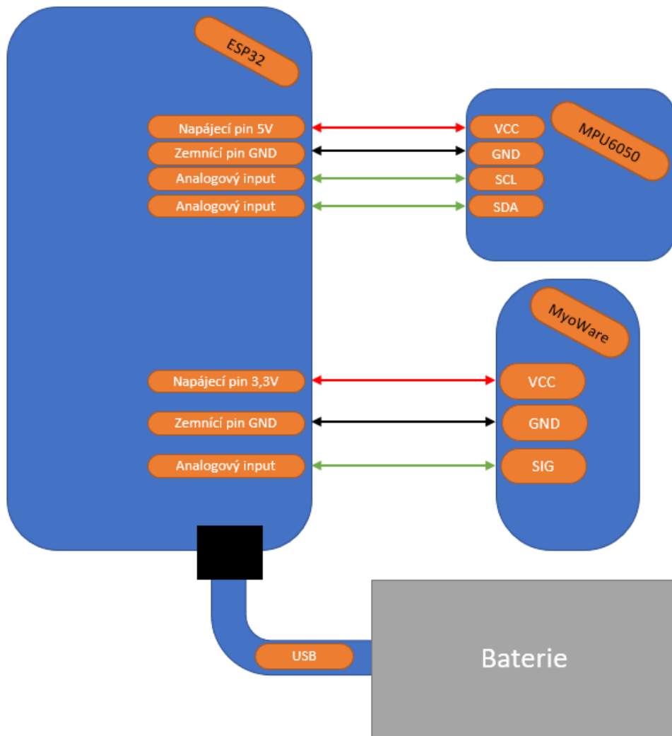
Obrázek 16 Schéma zapojení
