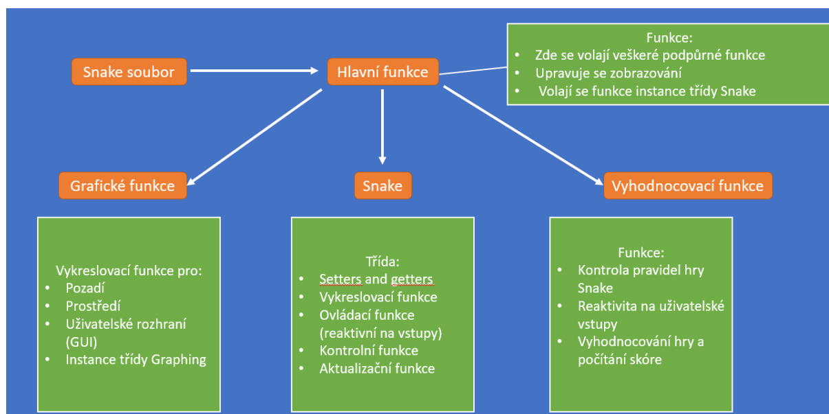
Obrázek 26 Schéma hry Snake
