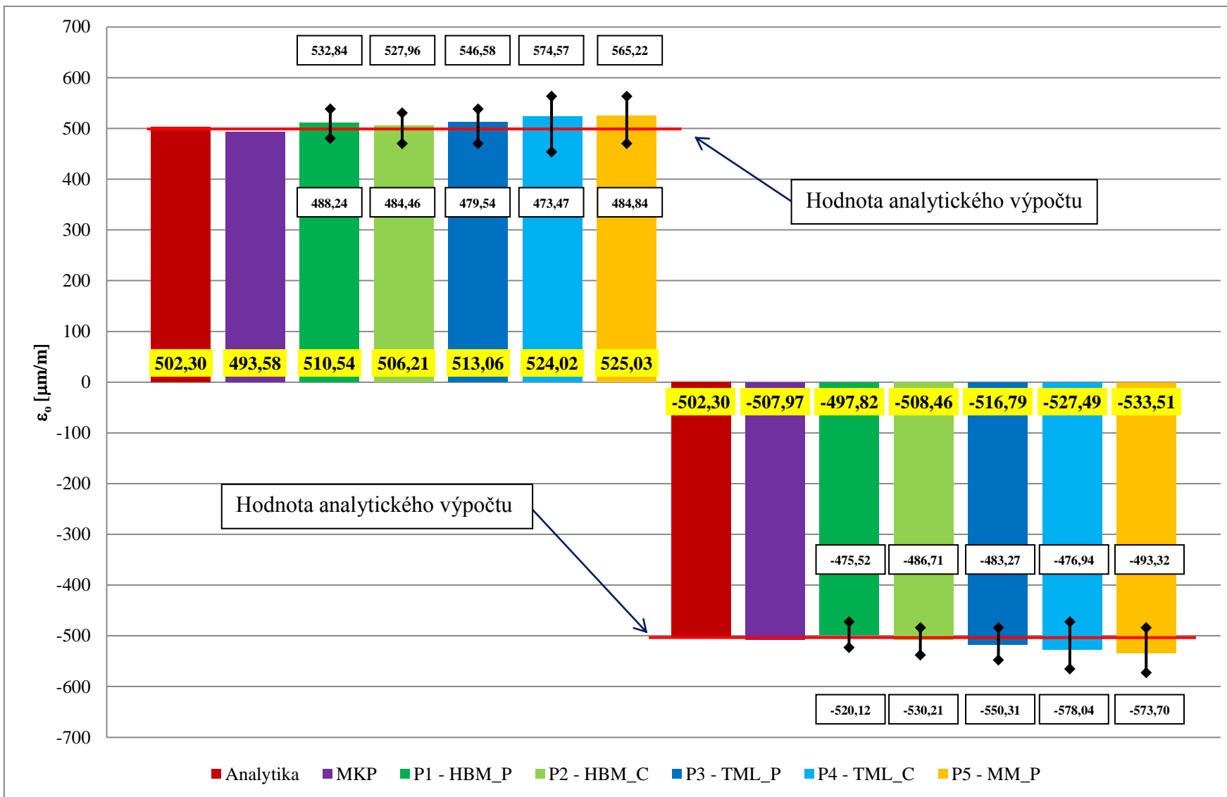
Graf P3.2: Výsledky, porovnání výpočtu a experimentu L = \pm 5 \text{ mm} se zahrnutím nejistoty měření U_{\text{cov}} , T = 90^\circ\text{C}
