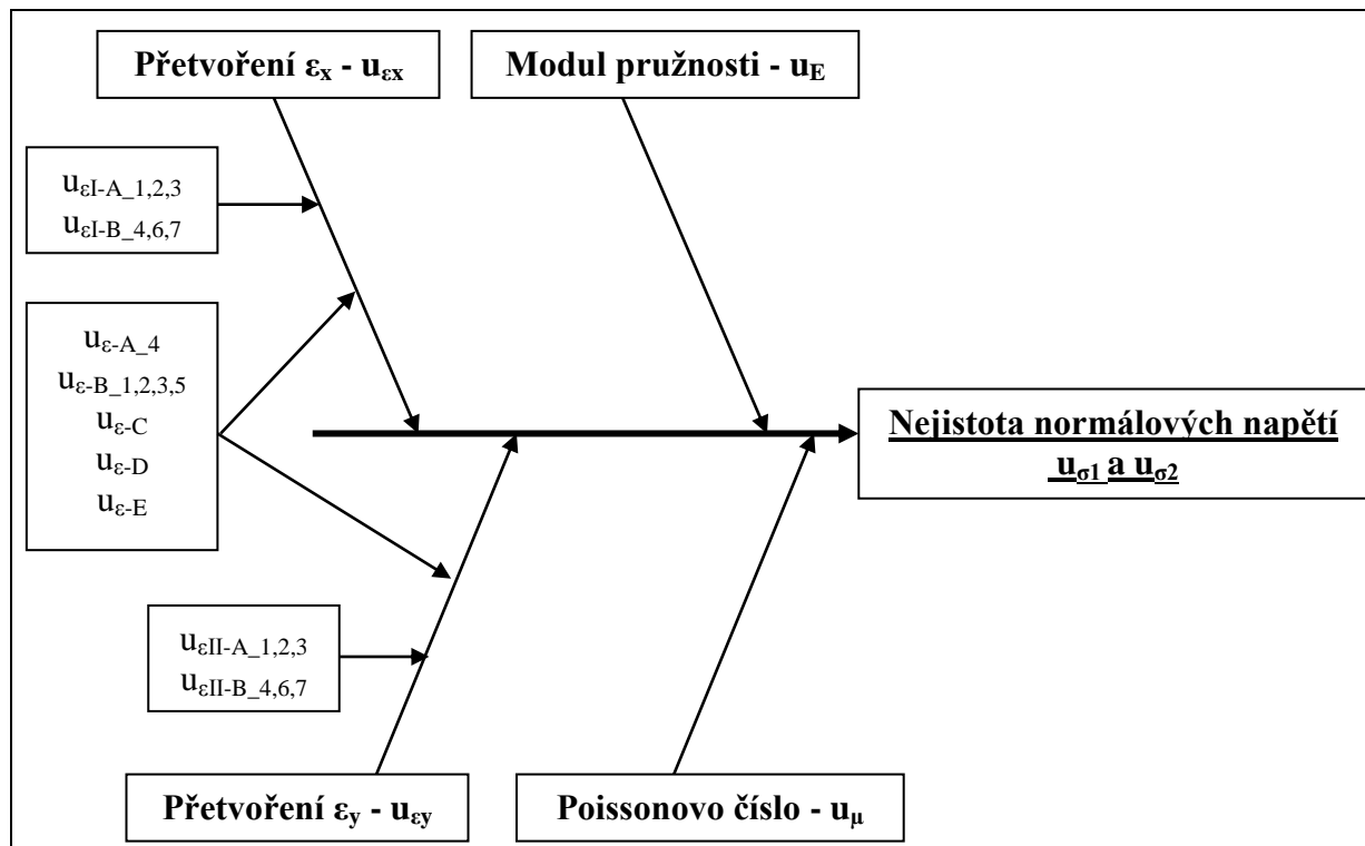
Obr. 5.9: Schéma zdrojů nejistot stanovených hlavních normálových napětí \sigma_1 a \sigma_2
