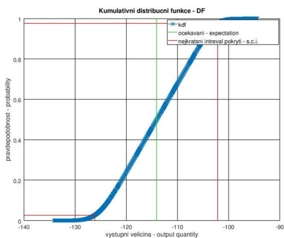
Graf 6.4: Kumulativní distribuční fce. L = -5 mm
