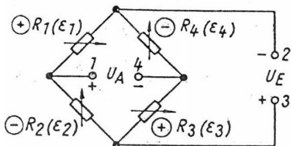
Obr. 3.3: Wheatstoneův můstek [17]
