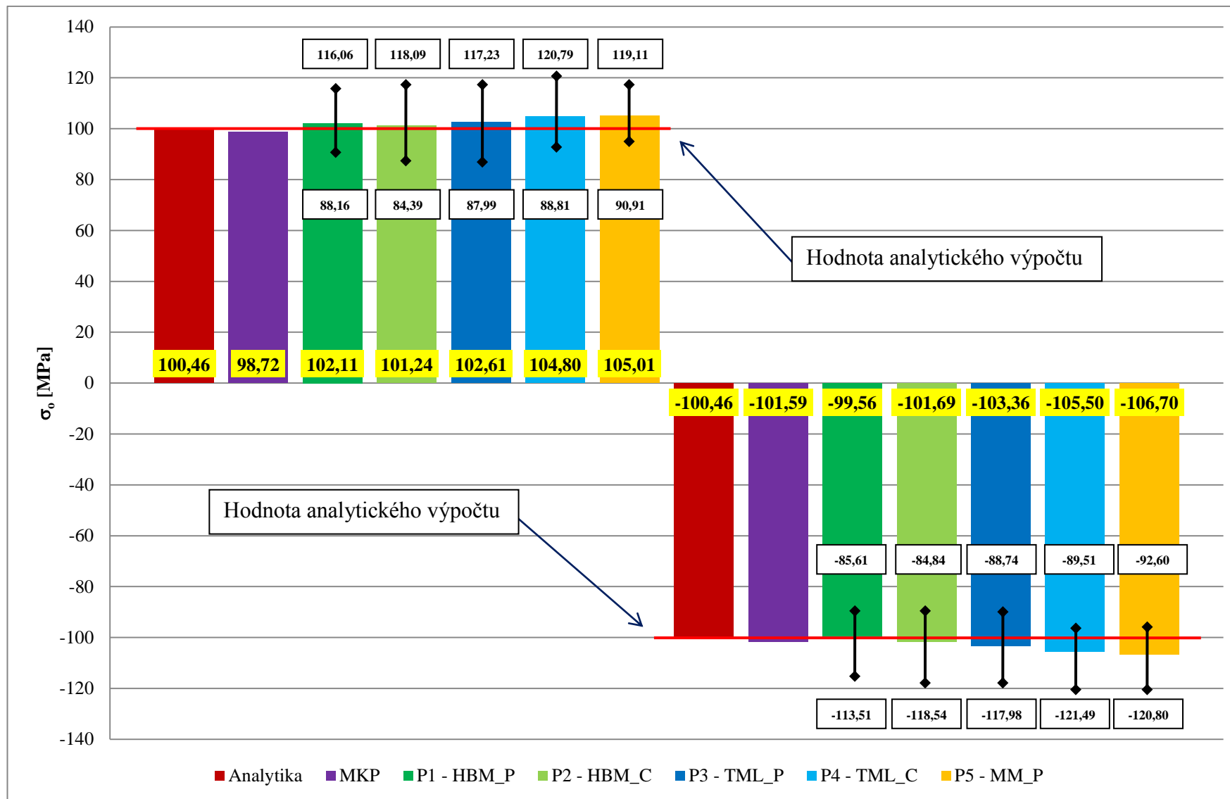
Graf P4.2: Výsledky, porovnání výpočtu a experimentu L = \pm 5 mm se zahrnutím nejistoty měření U_{\sigma\sigma} , T = 90^\circ\text{C}
