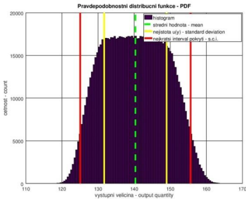
Graf 5.5: Fce. hustoty pravděpodobnosti \sigma_2
