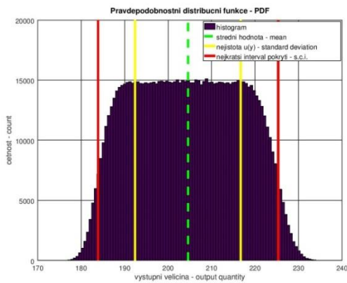
Graf 5.3: Fce. hustoty pravděpodobnosti \sigma_1
