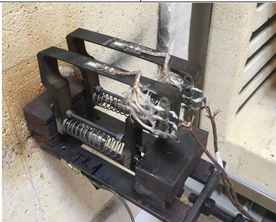
Obr. 6.9: Extenzometr P5 (MM-Vishay) umístěná v experimentálním zařízení (v peci)
