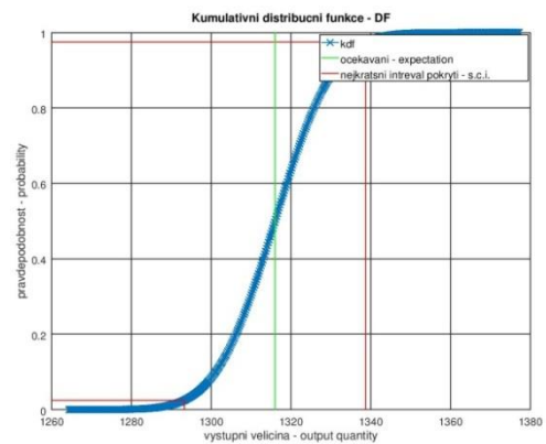
Graf 5.8: Kumulativní distribuční fce. \varepsilon_I
