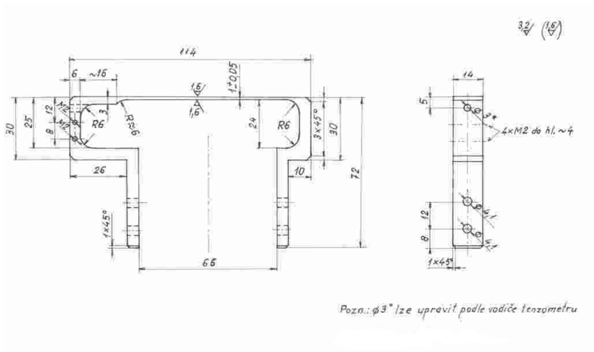
Obr. 6.2: Detail tělesa hrotového snímače posuvu
