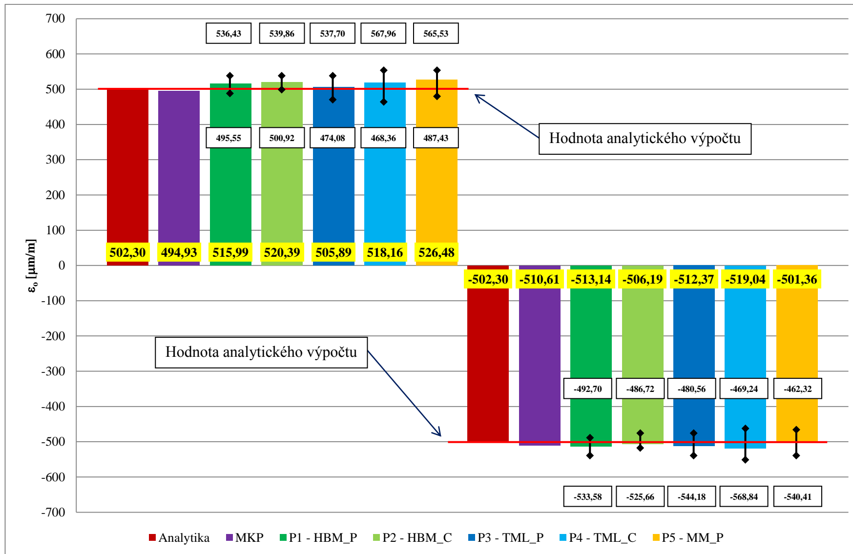
Graf P3.1: Výsledky, porovnání výpočtu a experimentu pro L = \pm 5 mm se zahrnutím nejistoty měření U_{\epsilon_0} , T = 20^\circ\text{C}
