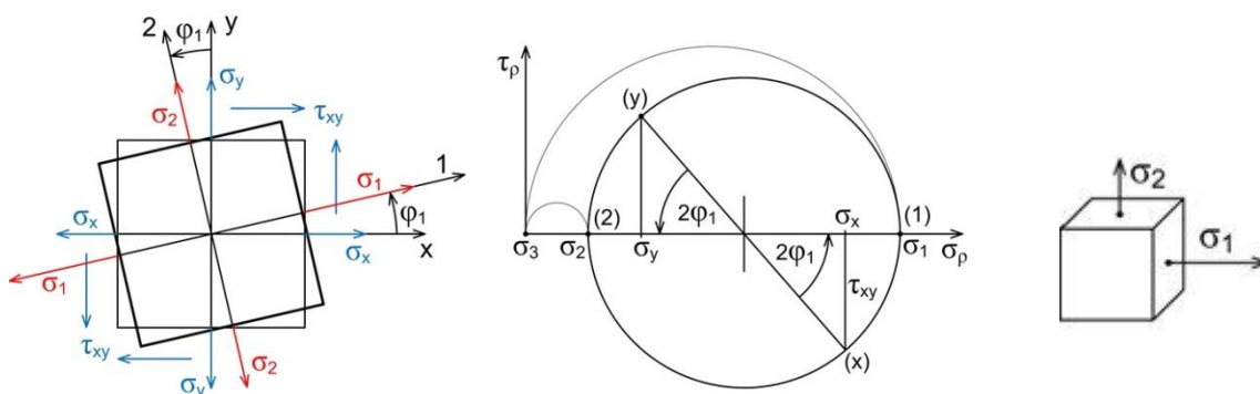
Obr. 4.2: Dvojosá napjatost [21]
