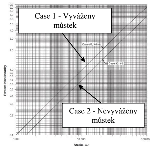
Obr. 3.4: Chyby nelinearity pro měřené \varepsilon [42]
