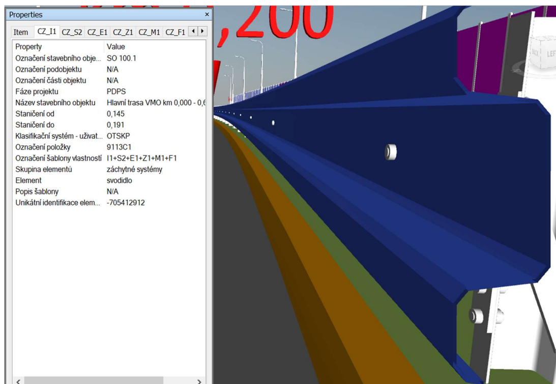
Obrázok 2: Ukážka už nakrmeného BIM modelu dátami (zvodidlom)
