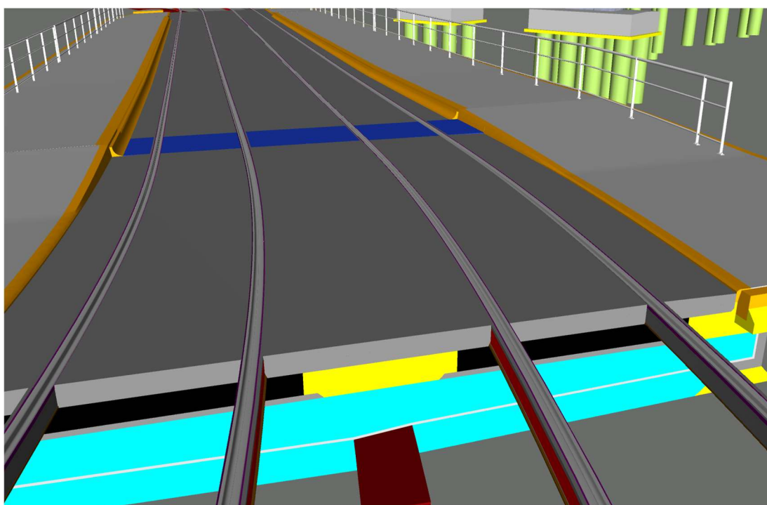
Obrázok 12: Ukážka z modelu z druhej strany zastávky, kde je vidieť rovnaký detail ako na obr.10 [Autor]
