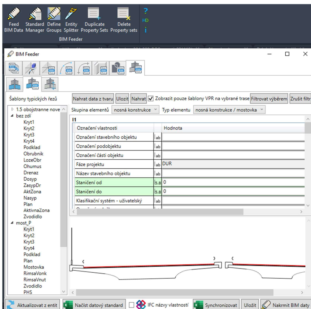
Obrázok 28: Ukážka prostredia BIM Feederu, vľavo úseky koridoru a kódy, vpravo už konkrétne vlastnosti a dole náhľad priečného rezu [Autor]
