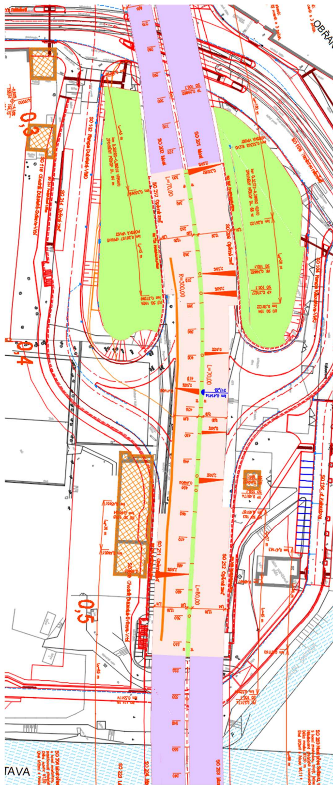
Obrázok 21: Situácia SO 100.1 medzi mostami cez Tomkovo námestie a cez rieku Svitavu, z dokumentácie PDPS
