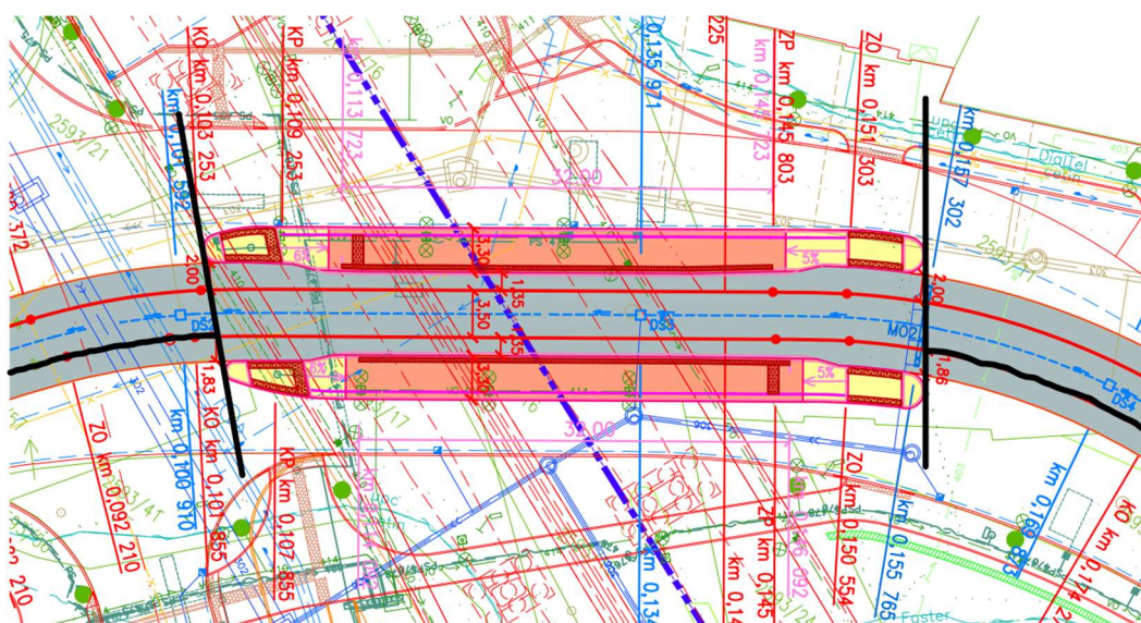
Obrázok 31: Situácia zastávky, hlavná osa električkovej trate v koridore Civilu (čierna) a priamka naznačujúca začiatok zastávky nie sú v pravom uhle, z dokumentácie PDPS [úpravy Autor]
