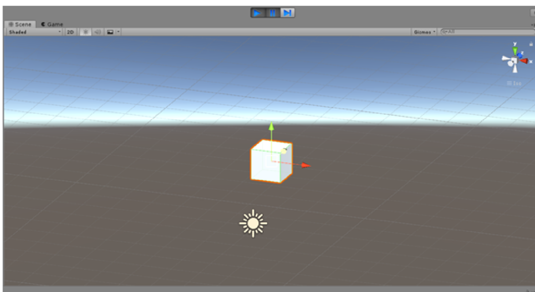
Obrázek 4.5: Pracovní plocha
