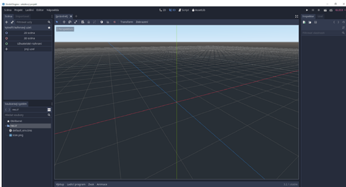
Obrázek 4.11: Prostředí Godot
