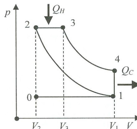
Obr. 6: Dieselův cyklus v p - V diagramu [7]
