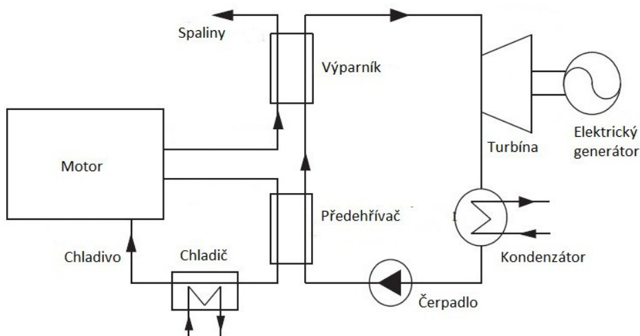
Obr. 20: RC cyklus s předehřívačem, převzato a upraveno ze zdroje [20]
